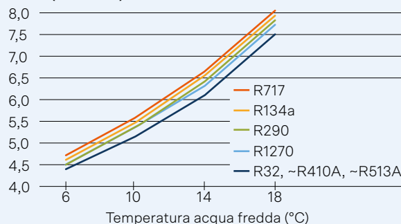
Efficienza energetica dei diversi fluidi refrigeranti EER ( t_c = 35\text{ °C} )*
