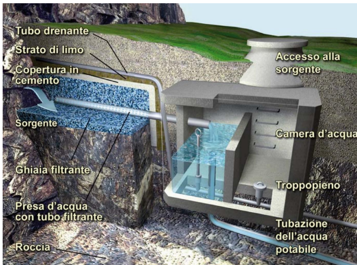
Figura 2 Captazione da sorgente: cunicolo drenante 5
