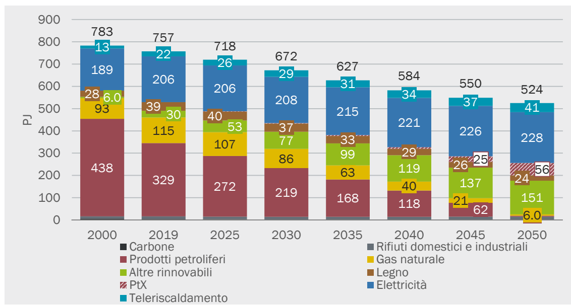
Figura 2: sviluppo del consumo di energia finale per vettore energetico
