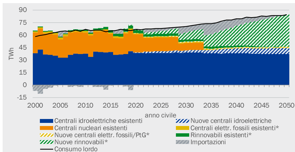
Figura 6: produzione di elettricità per tecnologia
