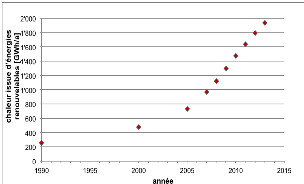
Figure 1: Evolution de l'utilisation de la géothermie au moyen de sondes et de pompes à chaleur sol/eau depuis 1990. (Source: OFEN: Statistiques suisses des énergies renouvelables. Edition 2013. Berne, septembre 2014)
