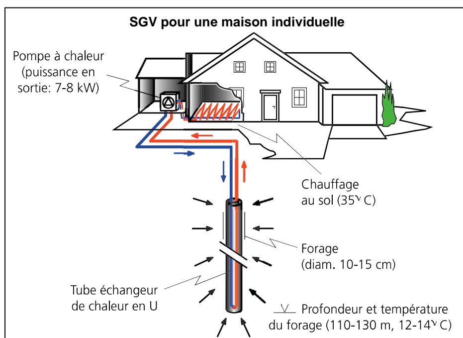
Figure 3: Illustration du système d'approvisionnement en chaleur d'une maison familiale par sonde géothermique et pompe à chaleur. (Source: www.geothermie.ch ).
