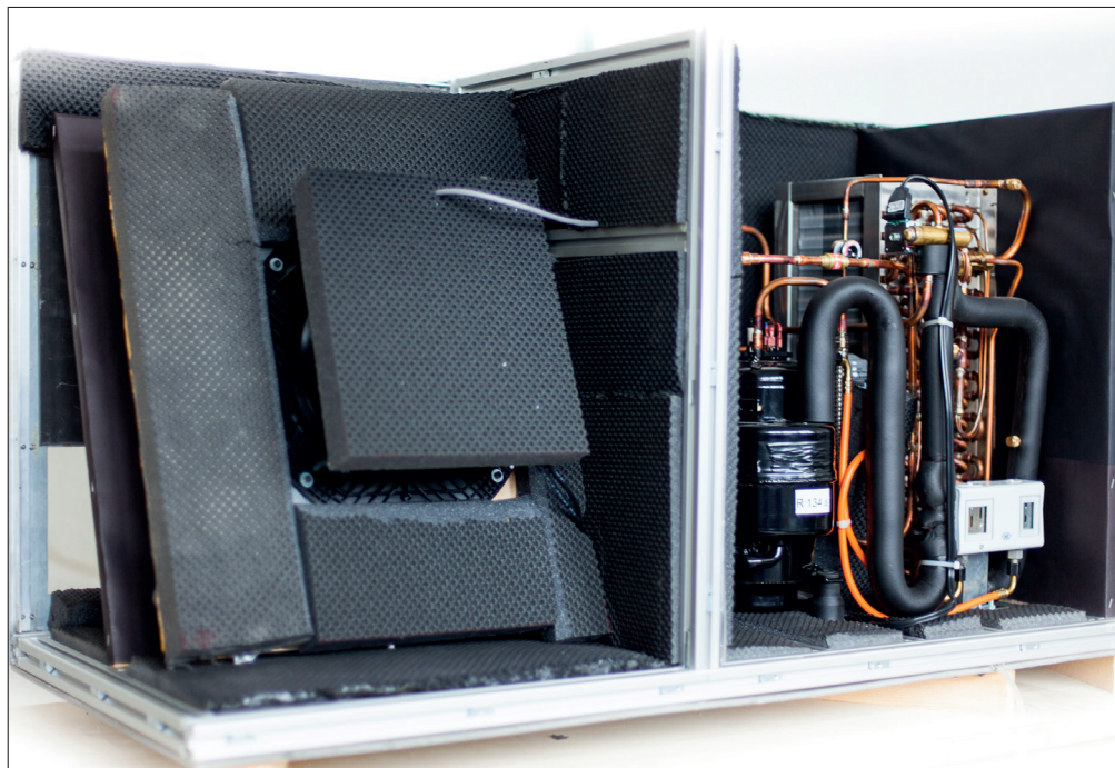
La thermopompe: à gauche, le côté air intérieur dans lequel des ventilateurs restituent la chaleur dans l'air de la pièce par le biais d'un échangeur thermique à lamelles (condensateur). A droite, le côté air extérieur dans lequel les composants habituels de la thermopompe (compresseur, évaporateur, collecteur, soupapes, etc.) sont disposés. PHOTO: AWTEC
