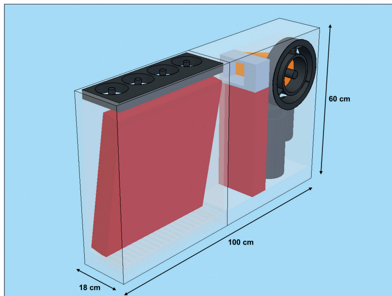
Représentation schématique du concept de la thermopompe: à gauche, le côté d'air intérieur (en haut, les ventilateurs pour le prélèvement de la chaleur dans l'air ambiant), à droite le côté air extérieur (avec l'admission et la sortie disposées de manière concentrique pour l'air extérieur).
