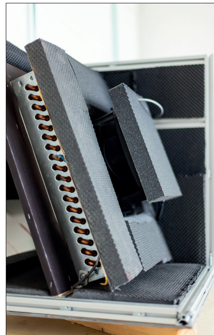
La chaleur est restituée dans l'air de la pièce avec des ventilateurs par le biais d'un échangeur thermique à lamelles (condensateur) sur le côté air intérieur. PHOTO: AWTEC
