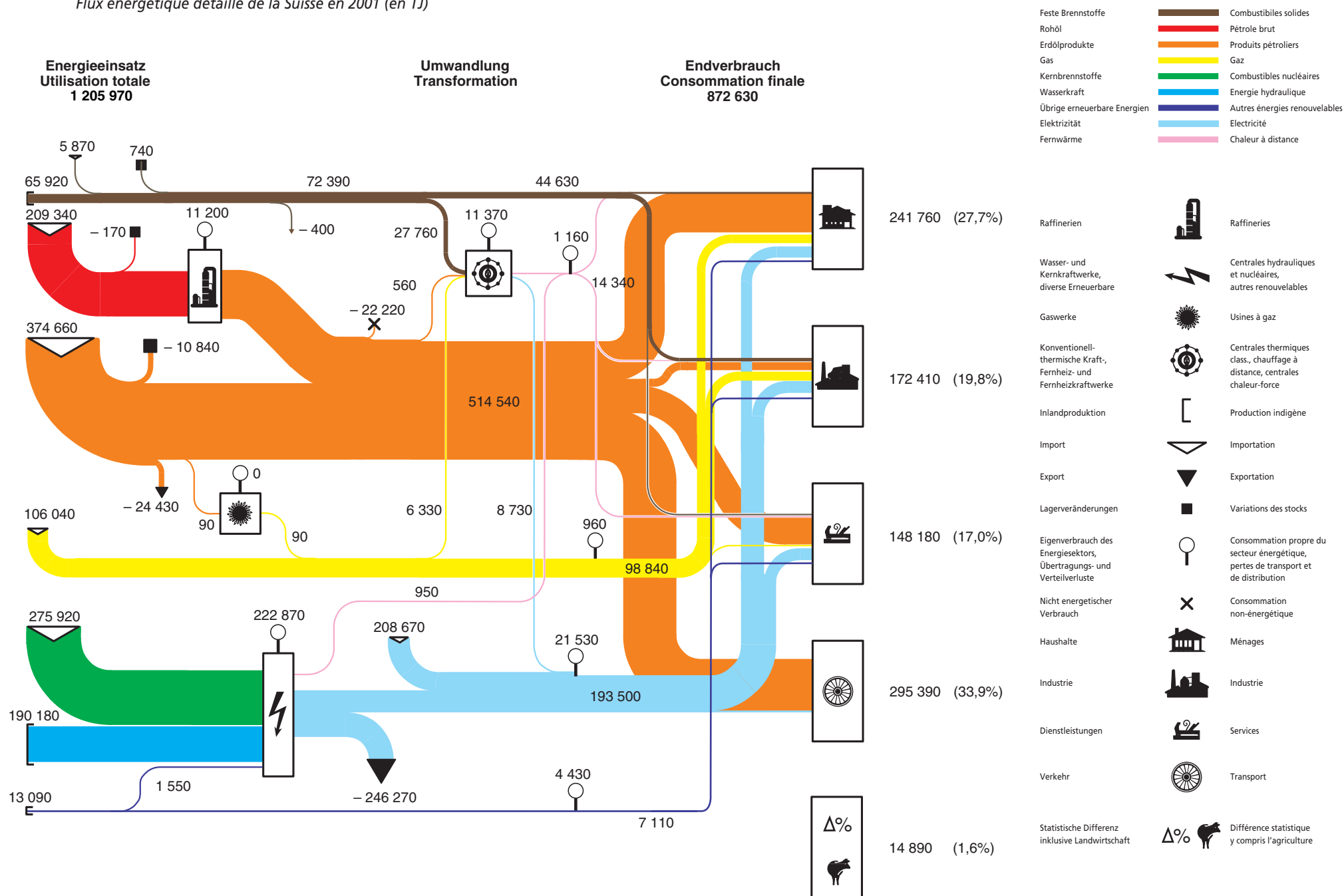
Fig. 5 Detailliertes Energieflussdiagramm der Schweiz 2001 (in TJ) Flux énergétique détaillé de la Suisse en 2001 (en TJ)
