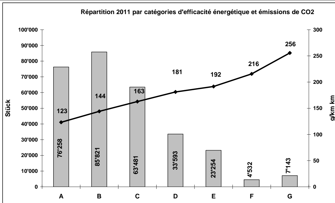
Graphique 5 Répartition 2011 par catégories d'efficacité énergétique et émissions de CO 2
