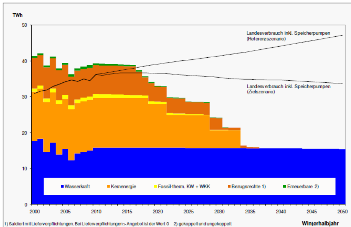
Grafik 46: Die Stromangebotsvarianten 1 und 2 Deckungsbedarf der Politikvarianten „Weiter wie bisher“ und „Neue Energiepolitik“, Winterhalbjahr in TWh el /a
