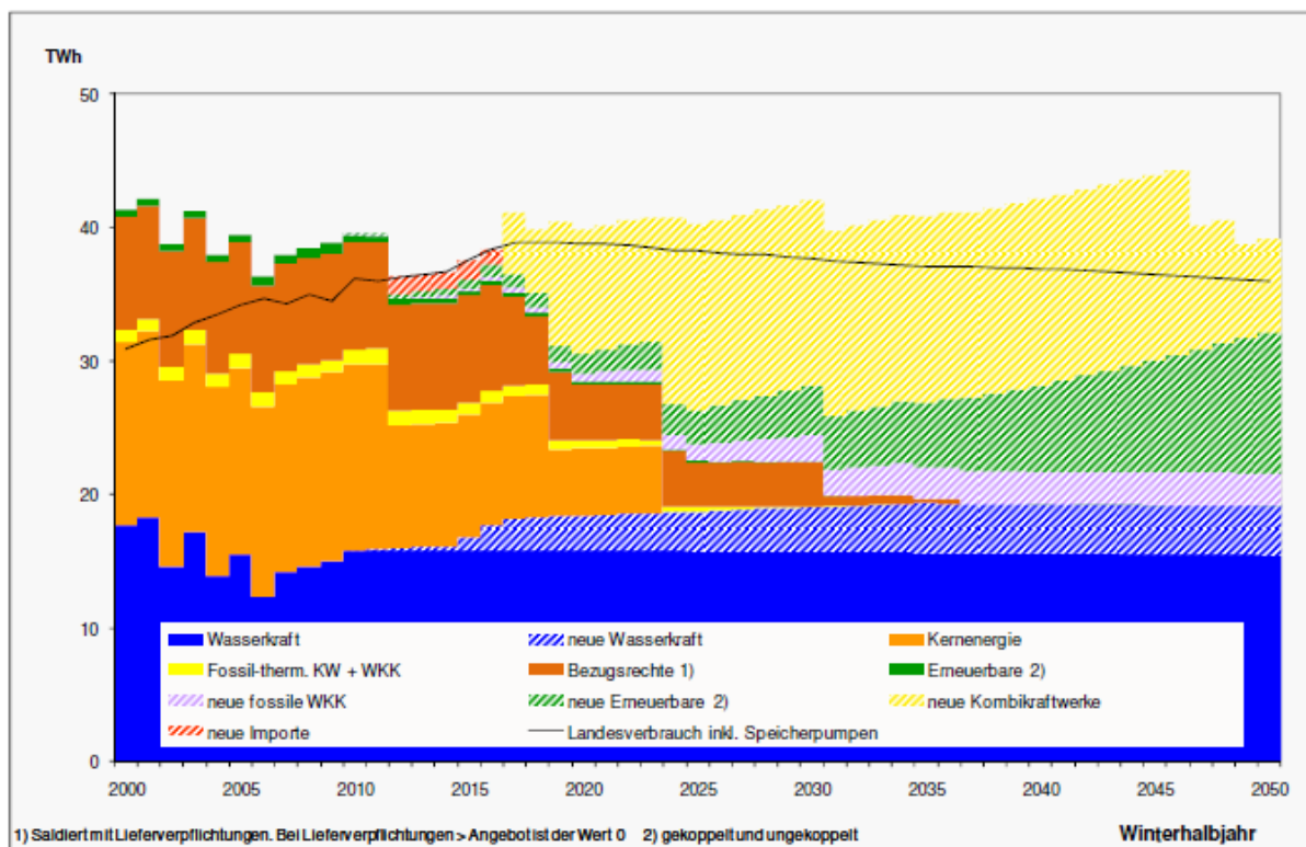
Grafik 32: Elektrizitätsangebot Bundesratsvariante 3 Variante C & E (Fossil-zentral und Erneuerbar), Szenario „Neue Energiepolitik“, Winterhalbjahr, 2000 - 2050, in TWh el /a
