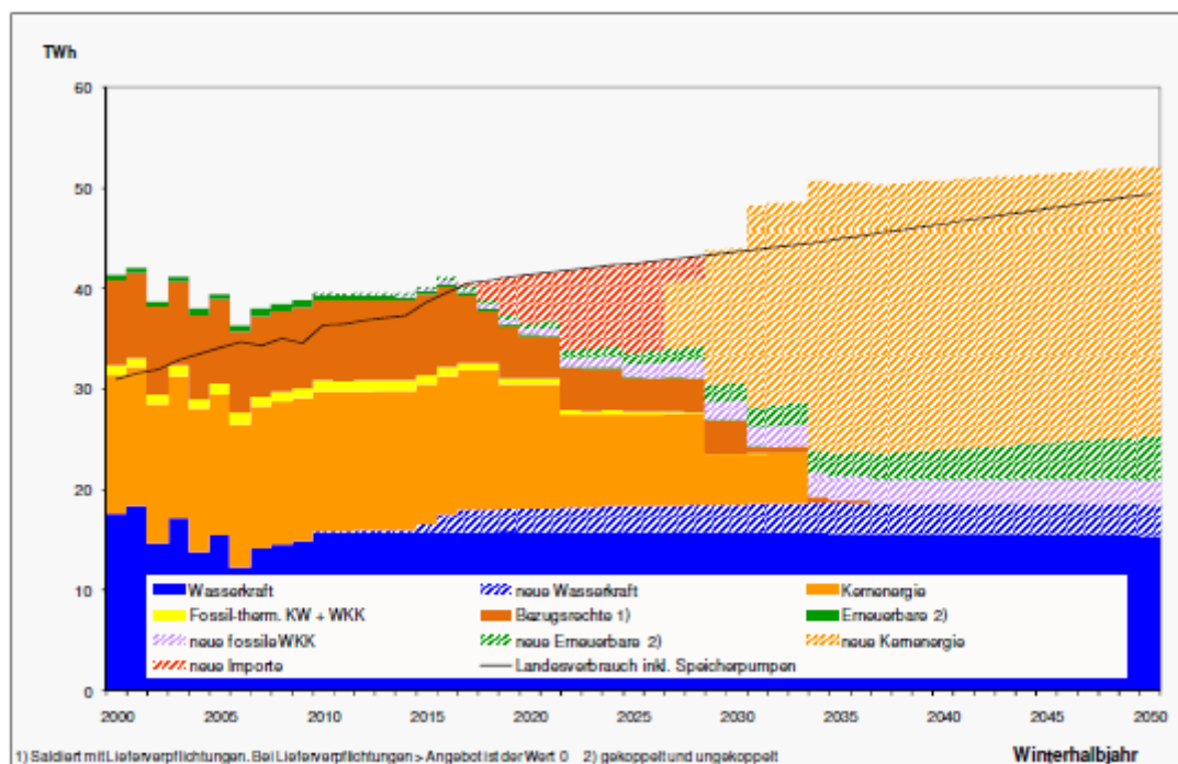
Grafik 11: Elektrizitätsangebot Bundesratsvariante 1 Variante A (Nuklear), Szenario „Weiter wie bisher“, Winterhalbjahr, 2000 - 2050, in TWh el /a
