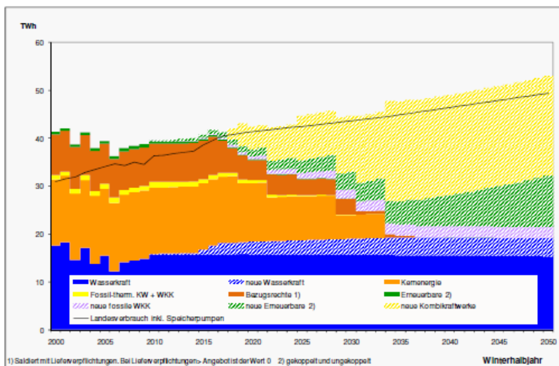
Grafik 15: Elektrizitätsangebot Bundesratsvariante 2 Variante C & E (Fossil-zentral und Erneuerbar), Szenario „Weiter wie bisher“, Winterhalbjahr, 2000 - 2050, in TWh e /a
