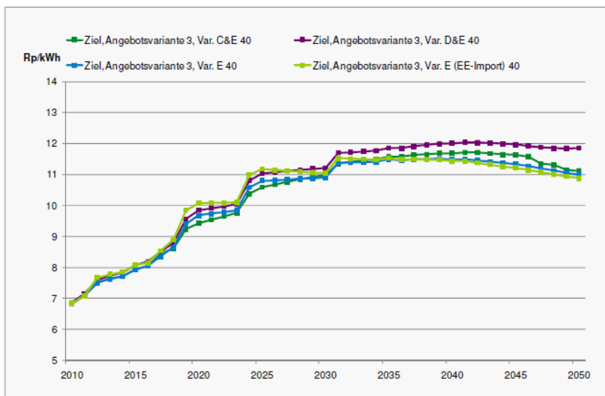
Grafik 44: Vergleich der Durchschnittskosten der Stromangebotsvarianten 3 des Bundesrats in der Politikvariante „Neue Energiepolitik“, in Rappen pro kWh el
