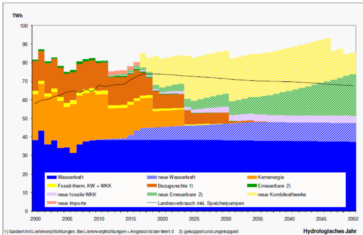
Grafik 31: Elektrizitätsangebot Bundesratsvariante 3 Variante C & E (Fossil-zentral und Erneuerbar), Szenario „Neue Energiepolitik“, hydrologisches Jahr, 2000 - 2050, in TWh el /a
