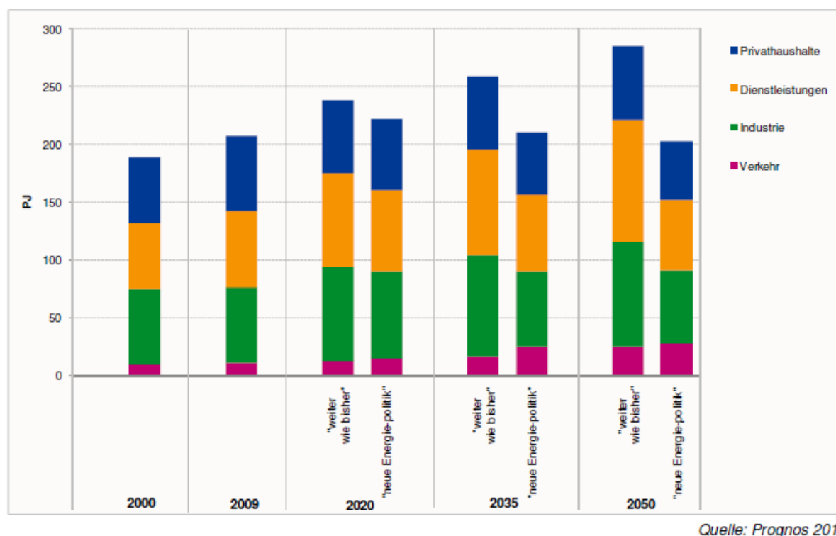
Figure R-5: Demande d'électricité par secteur (PJ)
