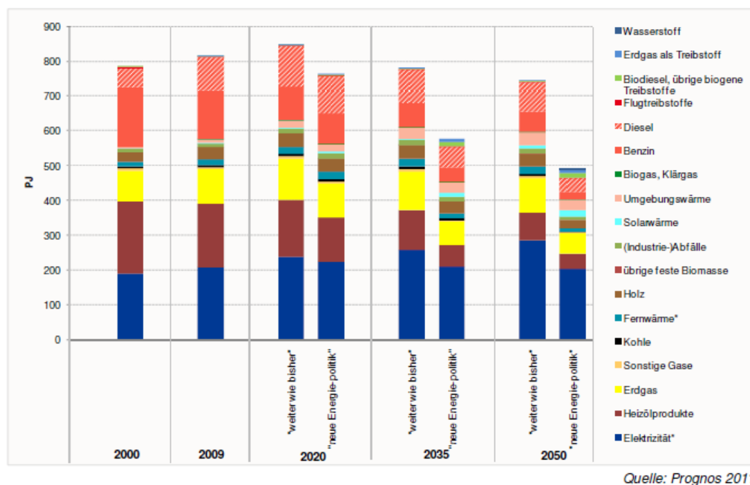
Figure R-1: Demande finale d'énergie par agent énergétique (PJ)
