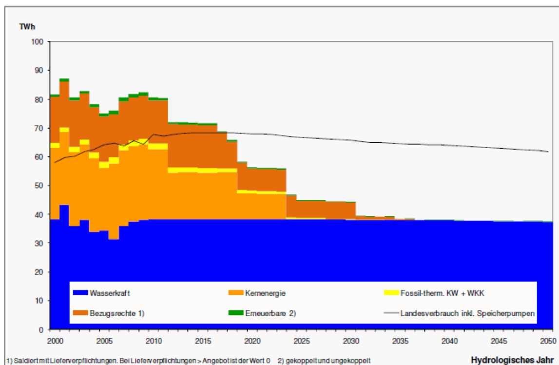
Figure R-7: Variante 3 de l'offre d'électricité, besoin à couvrir avec le scénario «Nouvelle politique énergétique», année hydrologique (TWh el /a)
