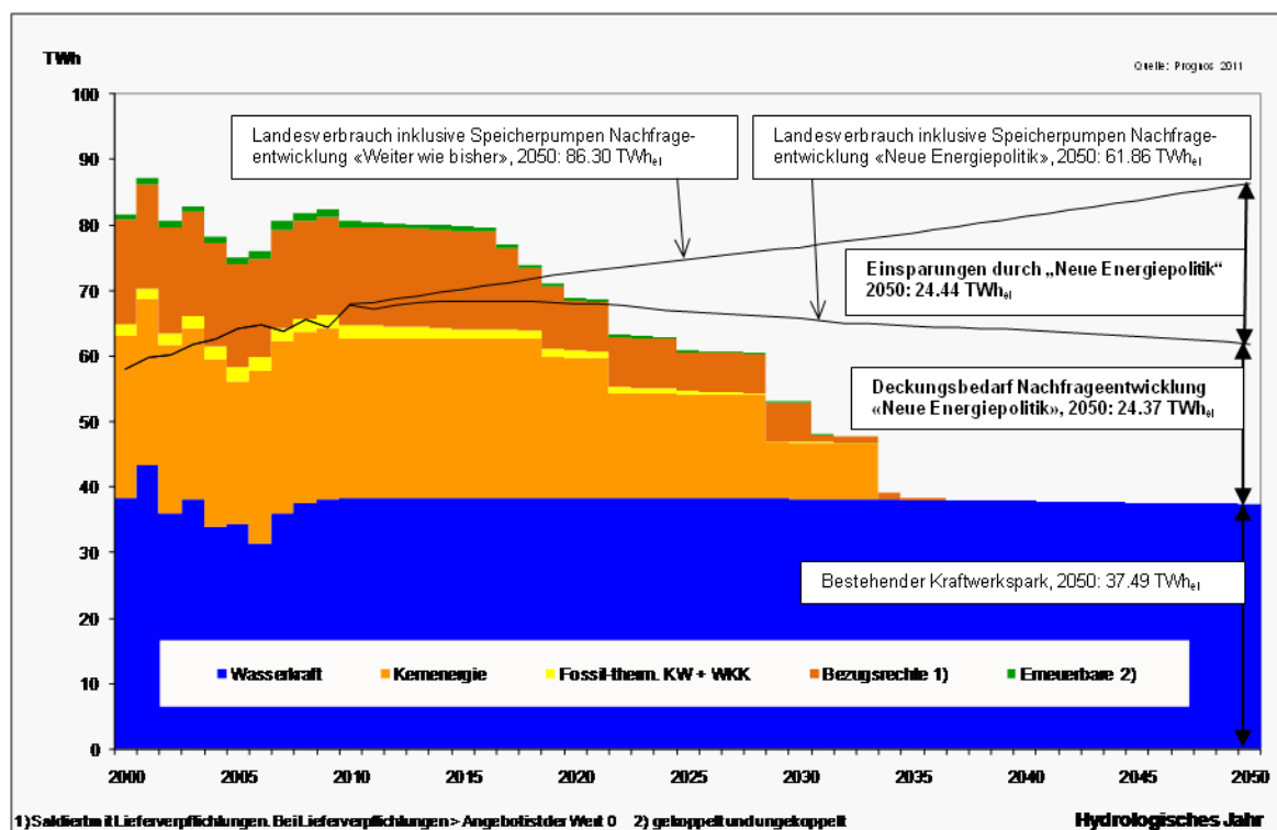
Figure R-6: Variantes de l'offre d'électricité 1 et 2, besoin à couvrir dans les options politiques „Poursuite de la politique actuelle“ et „Nouvelle politique énergétique“, année hydrologique (TWh el /a)
