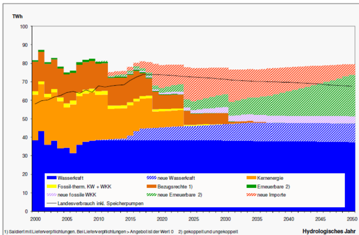
Grafik 35: Elektrizitätsangebot Bundesratsvariante 3 Variante E (Erneuerbar), Szenario „Neue Energiepolitik“, hydrologisches Jahr, 2000 - 2050, in TWh el /a
