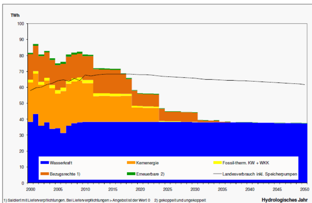
Grafik 47: Die Stromangebotsvarianten 3 Deckungsbedarf der Politikvarianten „Neue Energiepolitik“, hydrologisches Jahr in TWh el /a
