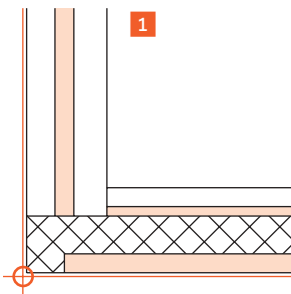
Isolation sous chape 4 cm
