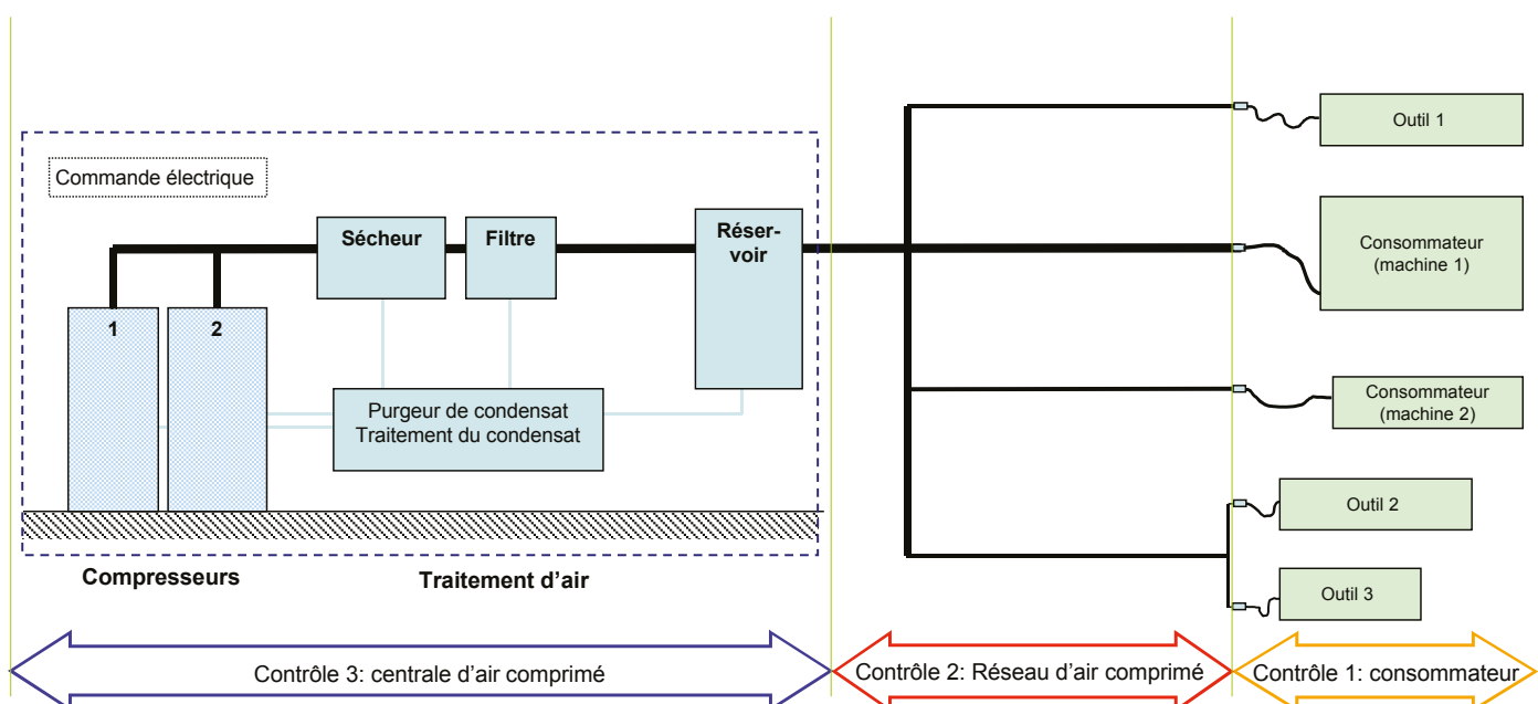
Illustration: Schéma d'une installation à air comprimé montrant les trois parties décrites dans le «contrôle en trois étapes»
