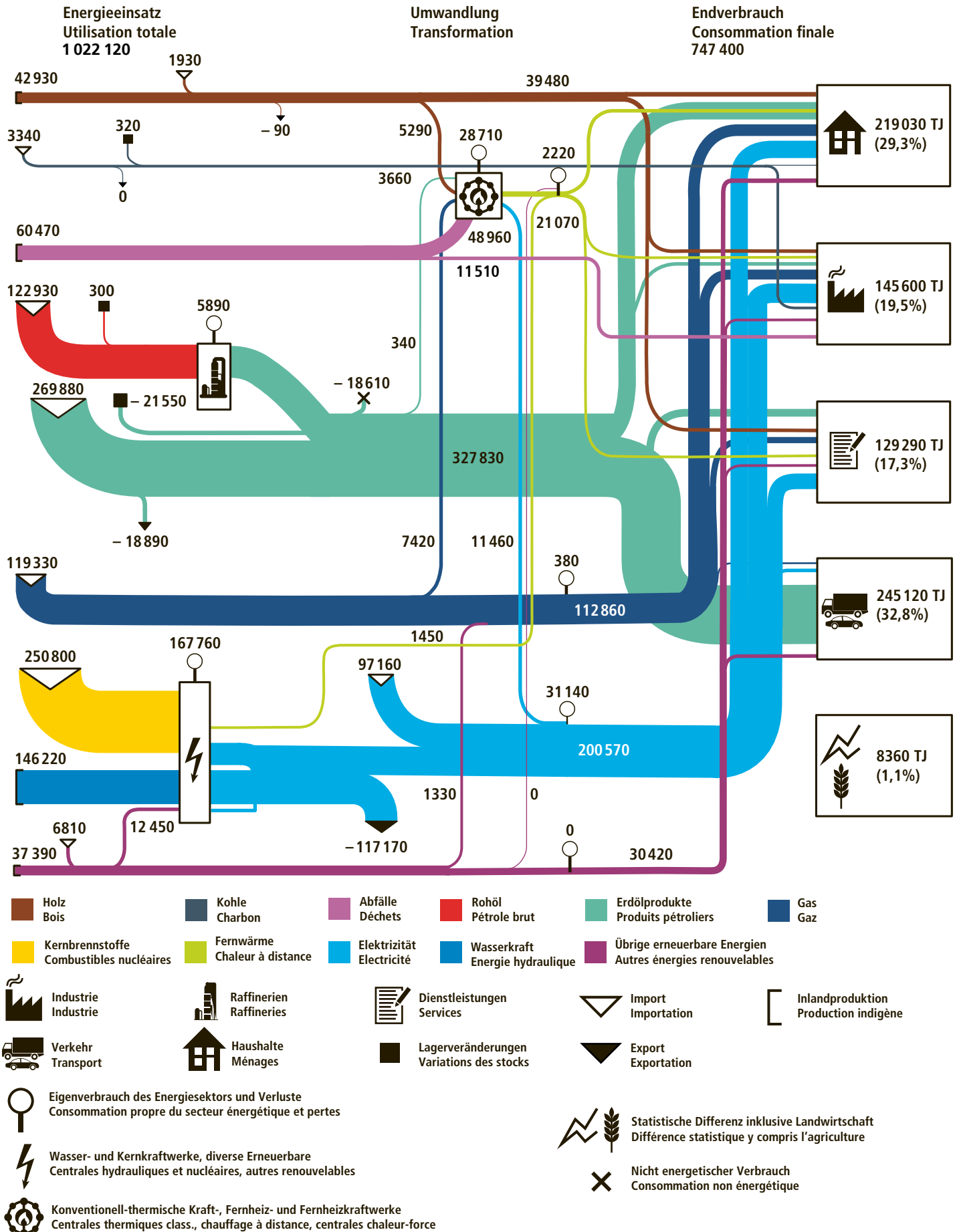
Fig. 5 Detailliertes Energieflussdiagramm der Schweiz 2020 (in TJ) Flux énergétique détaillé de la Suisse en 2020 (en TJ)
