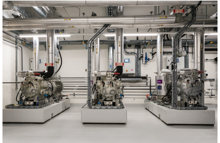
Deux compresseurs basse pression (à gauche, au centre) assurent le refroidissement des processus chez le fournisseur pharmaceutique Bachem AG à Bubendorf (BL). Le compresseur haute pression (à droite) utilise la chaleur résiduelle de la production de froid pour l'approvisionnement en chaleur de chauffage et en eau chaude. Photo: eicher+pauli Liestal AG
