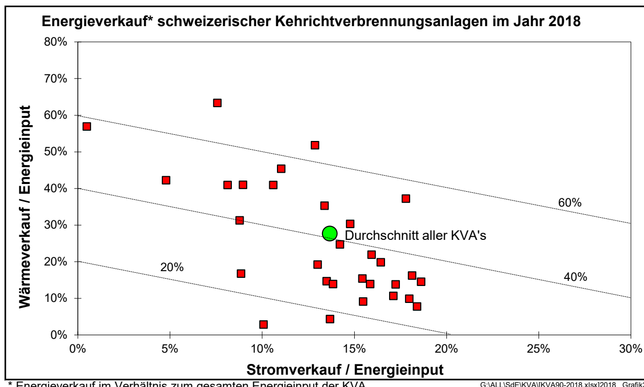
Bild 7.1d Energieverkaufs-Benchmark schweizerischer KVA (Jahr 2018)
