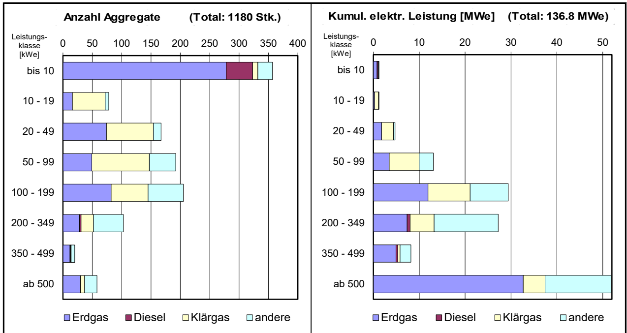
Bild 6.1f Ende 2018 in Betrieb stehende Klein-WKK-Aggregate, geordnet nach Leistungsklassen und nach Energieträgern
