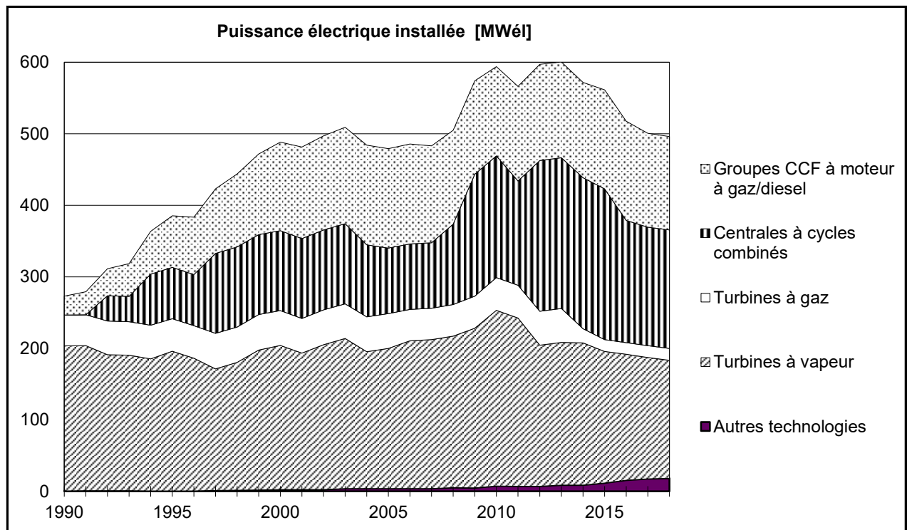
Figure 1.2 Evolution de la puissance électrique des installations à CCF selon leur type
