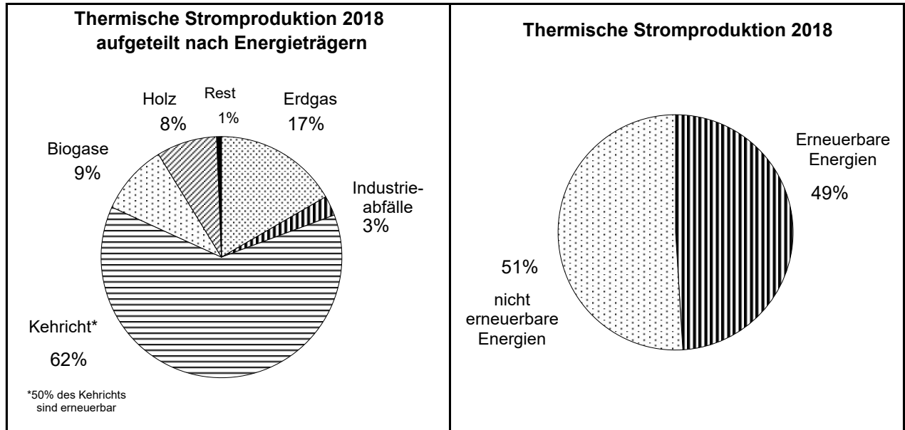
Bild 1.4 Aufteilung der thermischen Stromproduktion des Jahres 2018 nach Energieträgern
