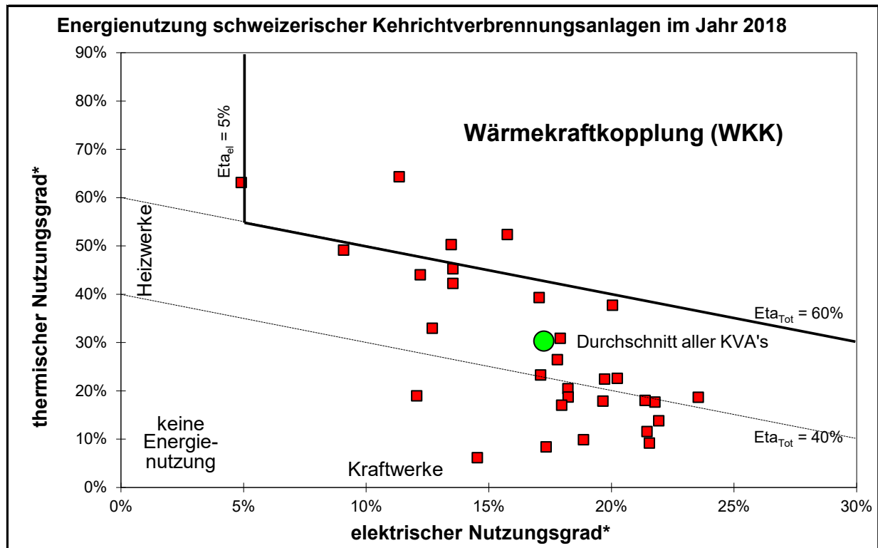
Bild 2.3 Jahresnutzungsgrade der schweizerischen Kehrichtverbrennungsanlagen im Jahr 2018
