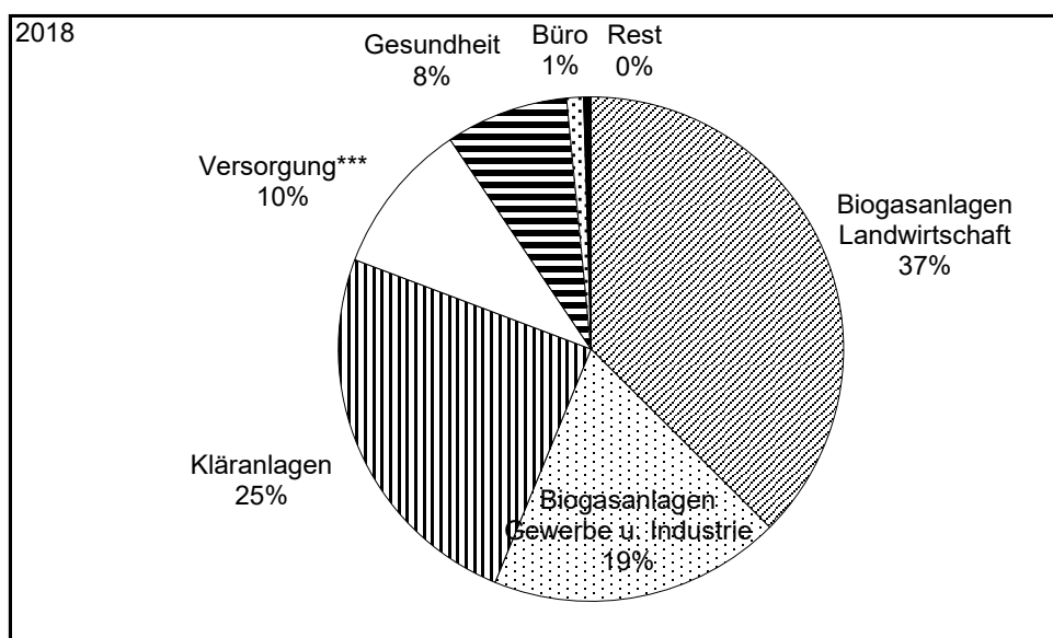
Bild 6.2d Neuinstallierte Klein-WKK-Leistung nach Einsatzgebieten (Jahr 2018)
