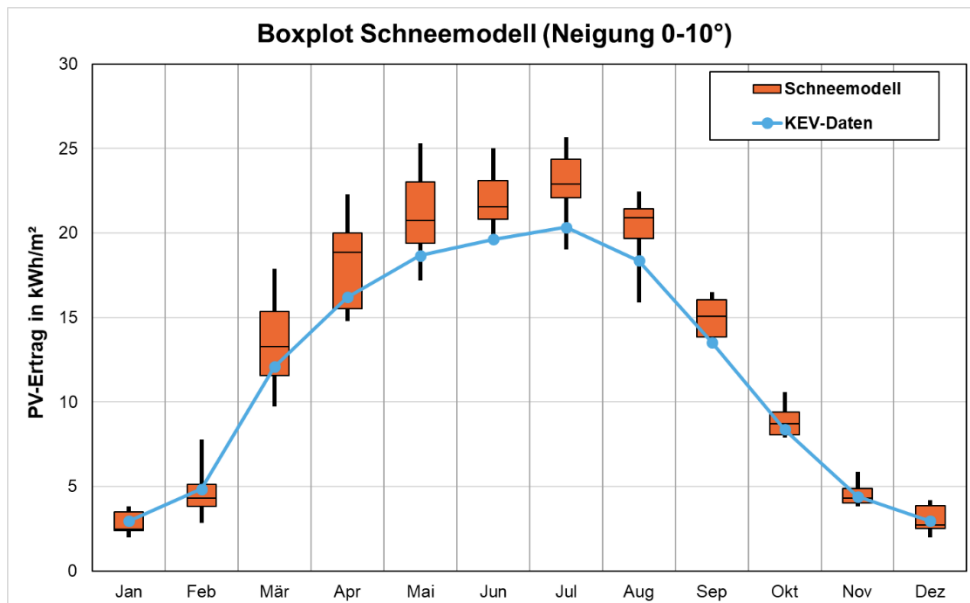
Abb. 19 Monatserträge des Schneemodells Neigung 0-10°, Validierung mit KEV-Anlagen.
