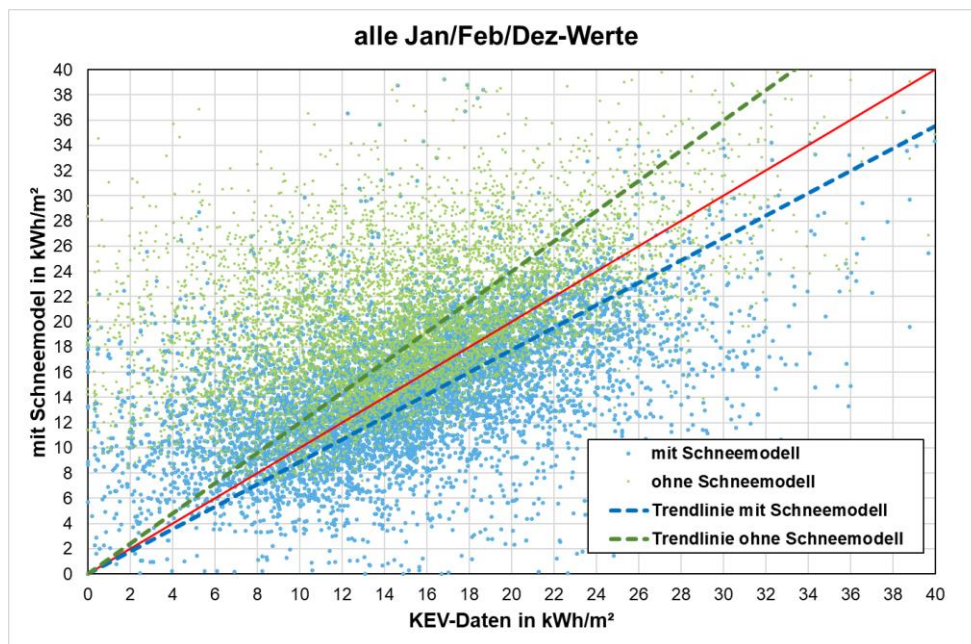
Abb. 17 Ertragsverlust durch Schneebedeckung. Diese Grafik umfasst die KEV-Anlagendaten aller Neigungen (0° bis 90°).
