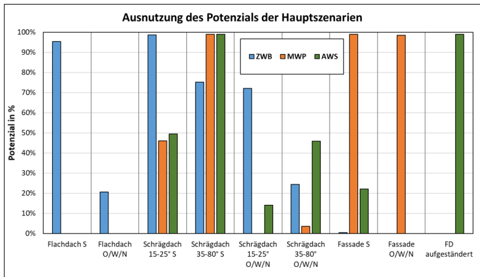
Abb. 4 Anteil der verwendeten Flächen am Gesamtpotenzial für die verschiedenen Hauptszenarien. Weil Sonnendach die meisten Flachdächer dem nördlichen Sektor zuordnet (hier der Kategorie "Flachdach O/W/N"), scheint die Kategorie "Flachdach S" stärker ausgeschöpft zu sein, als sie es in Wirklichkeit ist.
