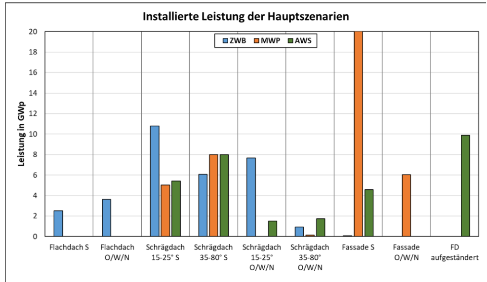
Abb. 5 Leistungsanteil verschiedener Flächen der Hauptszenarien. Weil die Flächen der Kategorie ZWB nicht eindeutig zugeordnet werden können, sind die Werte nur bedingt vergleichbar.
