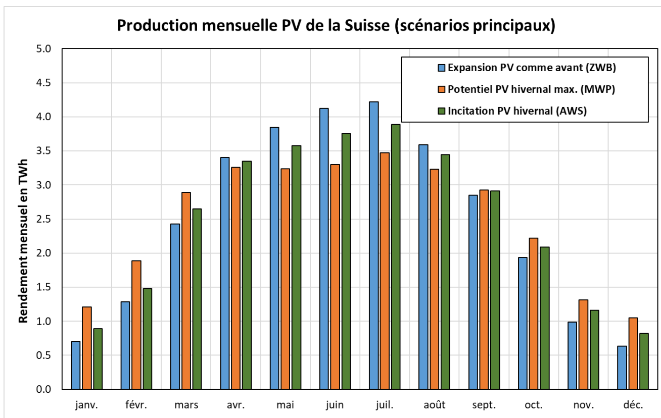
Abb. 2 Production mensuelle pour trois scénarios.
