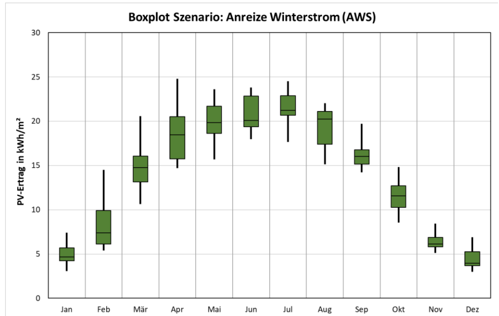
Abb. 10 Anreize Winterstrom (AWS), Boxplot. Die Bandbreite der Werte beruht auf den jährlichen Schwankungen der Einstrahlung.
