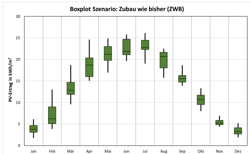
Abb. 8 Zubau wie bisher (ZWB), Boxplot. Die Bandbreite der Werte beruht auf den jährlichen Schwankungen der Einstrahlung.
