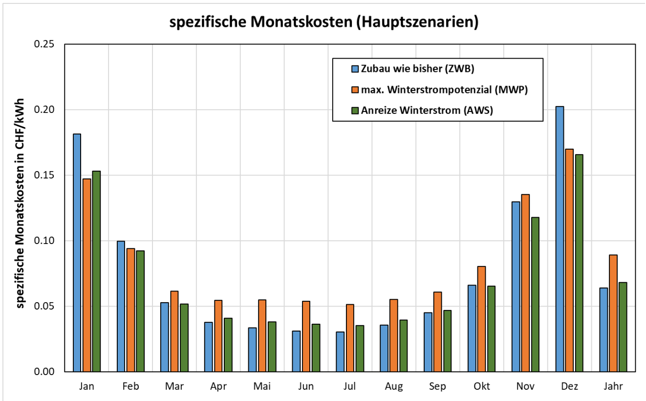
Abb. 13 Monatliche Stromgestehungskosten für die drei Hauptszenarien. Annahme: Jeder Monat wird 1/12 der Investitionskosten zugeschrieben.
