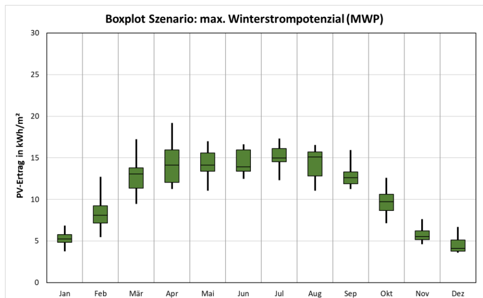
Abb. 9 Maximales Winterstrompotenzial (MWP), Boxplot. Die Bandbreite der Werte beruht auf den jährlichen Schwankungen der Einstrahlung.
