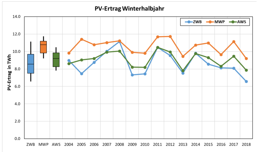
Abb. 12 Energieertrag des Winterhalbjahrs (Summe) der Jahre 2004 bis 2018.
