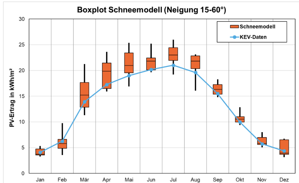
Abb. 21 Monatserträge des Schneemodells Neigung 15-60°, Validierung mit KEV-Anlagen.
