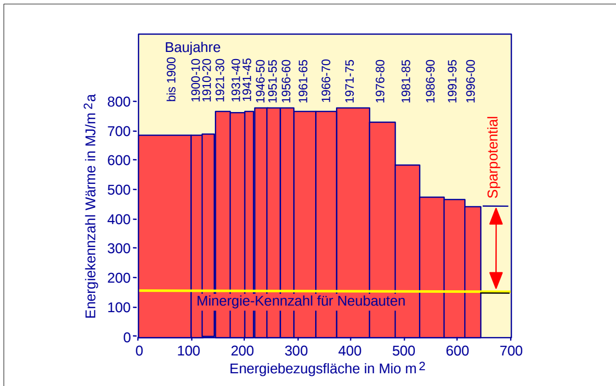
Figur 1: Die Graphik zeigt die im Kanton Zürich gebaute Wohnfläche mit dem zugehörigen spezifischen Energieverbrauch für Heizung und Warmwasser. Ab 1940 entspricht jedes Feld dem Energieverbrauch von Bauten einer 5-jährigen Bauperiode.
