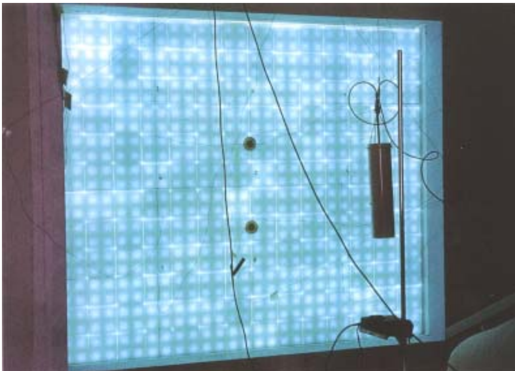
Figur 2: Messungen im Solarprüfstand der EMPA haben gezeigt, dass die mit Parafinspeicher bestückte transluzente Fassade (Architekt D. Schwarz [32]) im Winter die Sonnenwärme gut einfängt, währenddem sie im Sommer einen guten Sonnenschutz bietet.
