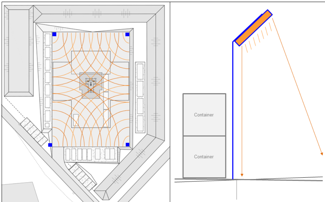
Fig. 5.8: Beispielhafte Ausleuchtung des Arbeitsbereichs für den Bohrplatz (Leuchte mit Wirkungsbereich).
