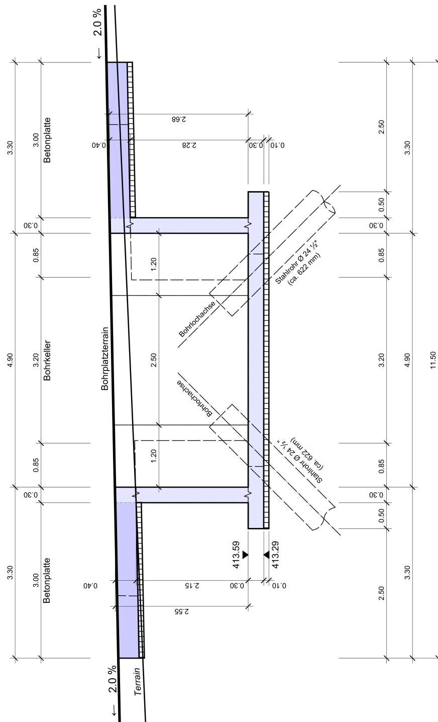
Fig. 5.5: Querschnitt des Bohrkellers (A-A) mit den Bohrrichtungen W und E und den entsprechenden Bohransatzpunkten (Lage des Schnitts vgl. Beilage 8).
