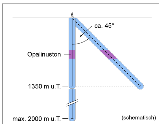
Fig. 7.1: Lage und Ausdehnung der möglichen Bohrfade der Sondierbohrungen Stadel 1 in Bezug auf die SMA- und HAA-Lagerperimeter mit Sicherheitsabstand von r = 50 m um die potenziellen Bohrfade.
