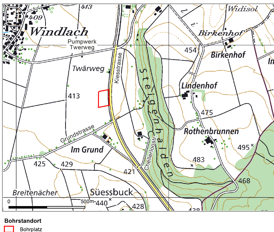
Fig. 5.1: Lage und Grösse des Standorts des Bohrplatzes Stadel 1.
