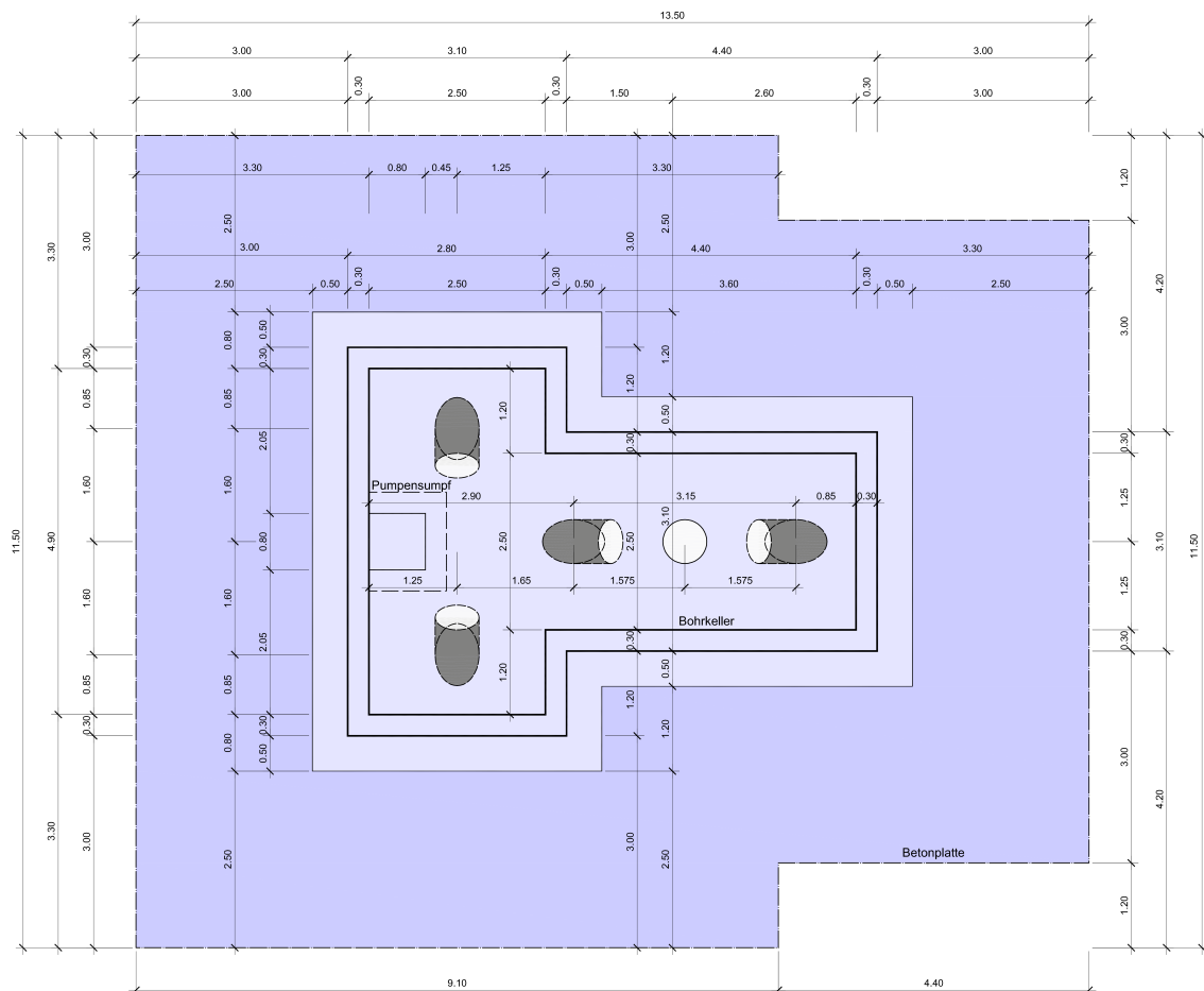
Fig. 5.3: Grundriss des Bohrkellers für fünf Bohrrichtungen.
