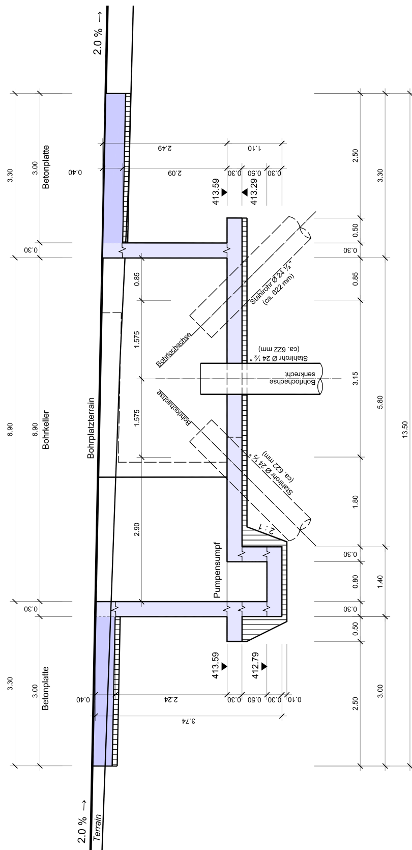
Fig. 5.4: Längsschnitt (B-B) des Bohrkellers mit den Bohrrichtungen N und S und den entsprechenden Bohransatzpunkten (Lage des Schnitts vgl. Beilage 8).
