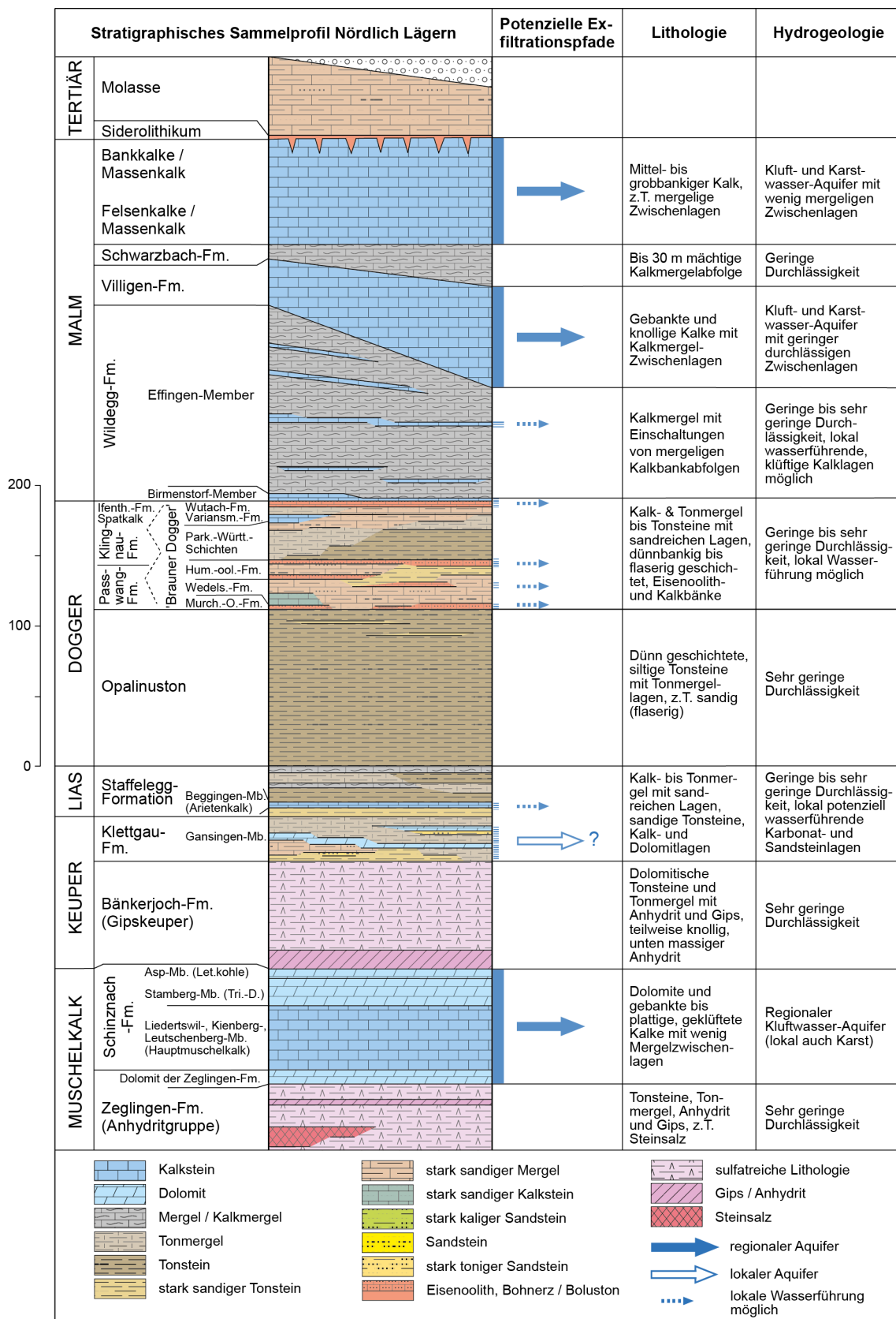
Fig. 2.1: Schematisches stratigraphisch-hydrogeologisches Sammelprofil für das Standortgebiet Nördlich Lägern (nach Nagra 2014b, Dossier II).
