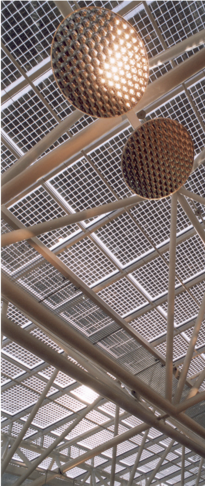
In Isolierglas integrierte PV-Zellen, welche der Migros Genossenschaftsbund im Jahr 2000 an seinem Hauptsitz am Limmatplatz in Zürich realisiert hat. Foto: energiebüro® ag / Zürich - für Solarkraftwerke
