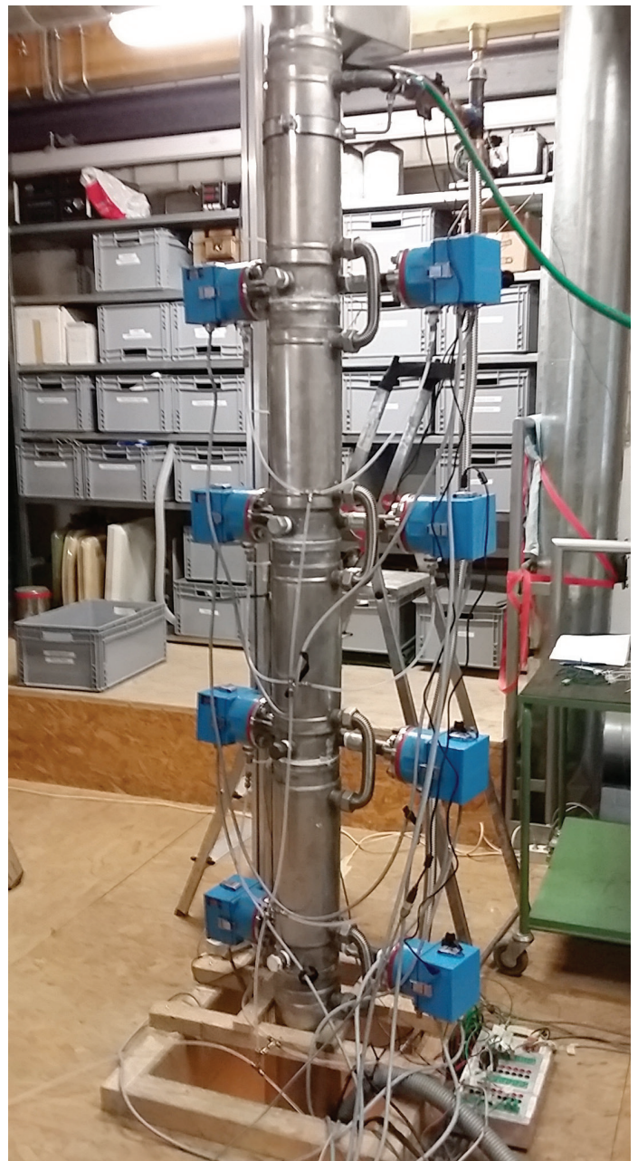
Der NOSMOG-Prototyp für Holzfeuerungen bis zu 70 kW Leistung, der im Zuge des jüngsten NOSMOG-Projekts im Forschungslabor des Ökozentrums in Langenbruck aufgebaut wurde. Mit den Messgeräten (blau) hat die Fachhochschule Nordwestschweiz in Windisch sogenannte Extinktionsmessungen durchgeführt, um den Prozess der Abgasreinigung besser zu verstehen. Foto: B. Salerno
