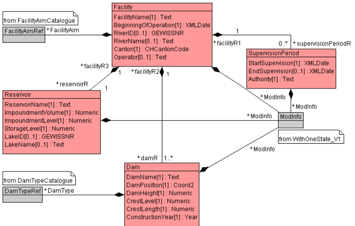
Abbildung 3: UML-Klassendiagramm Thema «DamsUnderSupervisionByCantonalGovernment_WithOneState»
