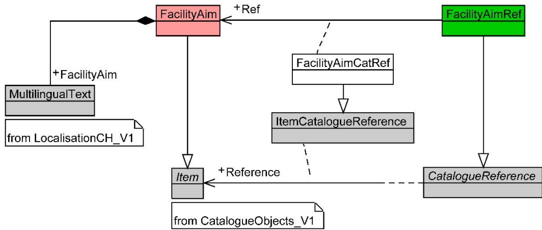
Abbildung 4: UML-Klassendiagramm Thema «FacilityAimCatalogue»
