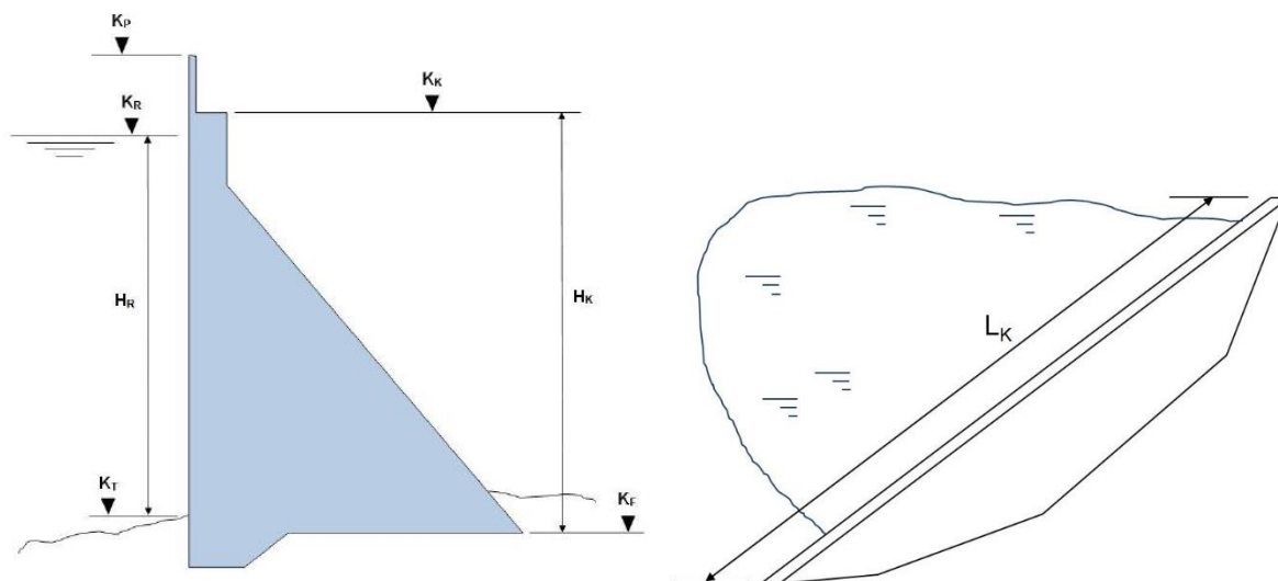
Abbildung 7: Schematische Darstellung eines Absperrbauwerks
