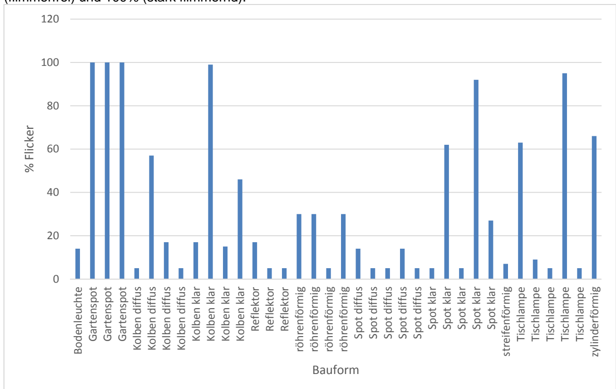
Fig. 4 Flickereigenschaften von LED (36 verschiedene LED)
