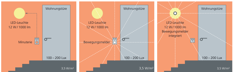
Minuterie (Zeitschaltuhr)
