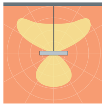
Pendelleuchte 20–100 W 1500–12000 lm*
