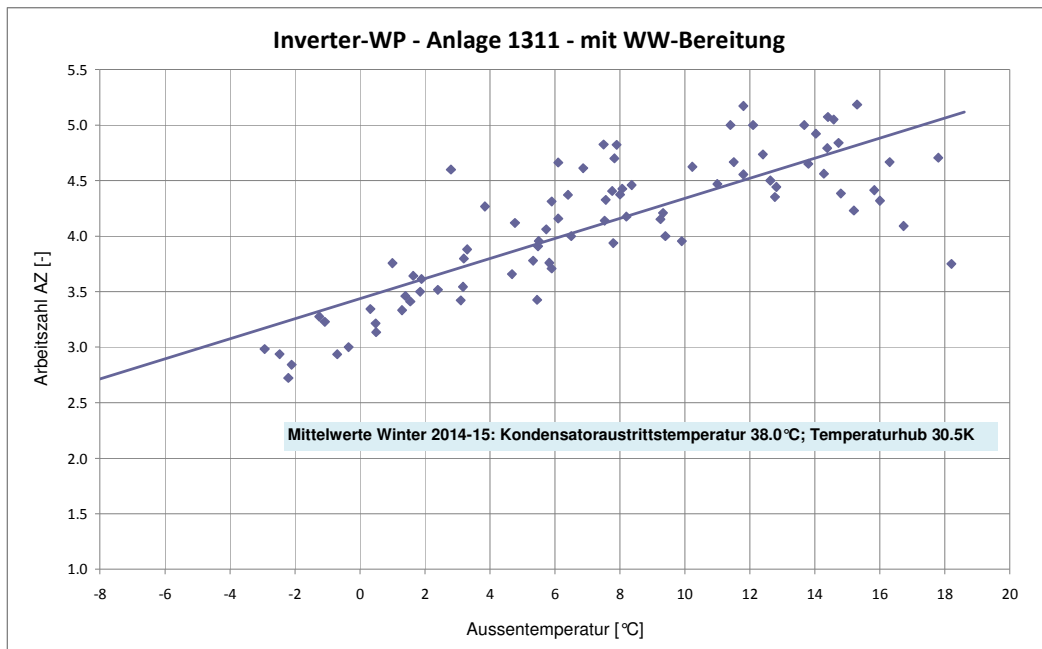
Abb. 48: Anlage 1311, Verlauf der Arbeitszahl versus Aussentemperatur im Winterbetrieb
