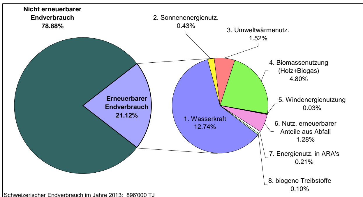
Bild 4.5 Endverbrauchsanteil der erneuerbaren Energien 2013 - Gliederung nach Technologien (grafische Darstellung der Werte gemäss Bild 4.4)
