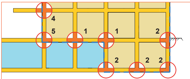
Abb.: Gebäudeschnitt mit Orten an denen Wärmebrücken/Erdbebensicherheits-Konflikte auftreten (Nummern entsprechen Wärmebrückentypen in der Tabelle)
