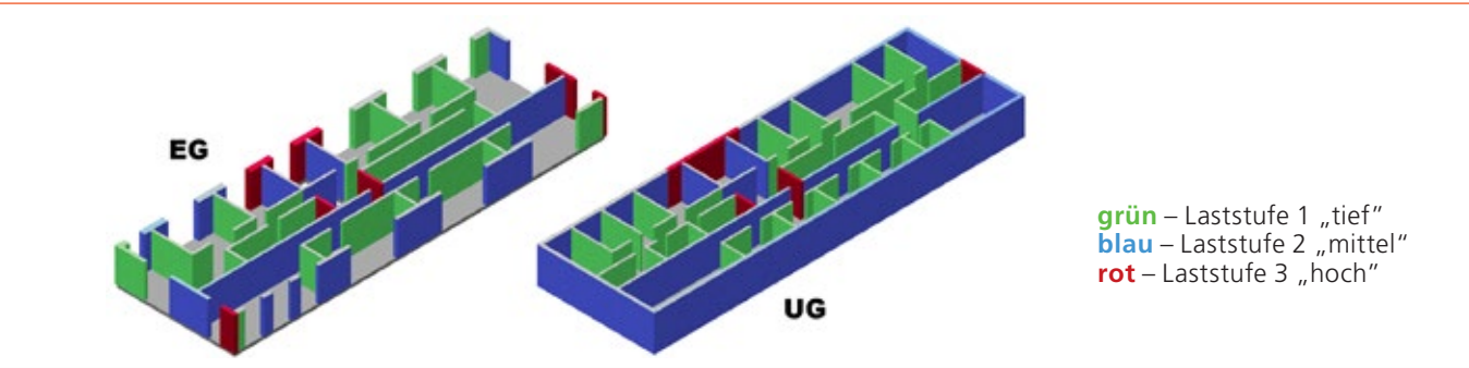
Abb.: Grundrisse Erd- und Untergeschoss des Referenzgebäudes mit Laststufen
