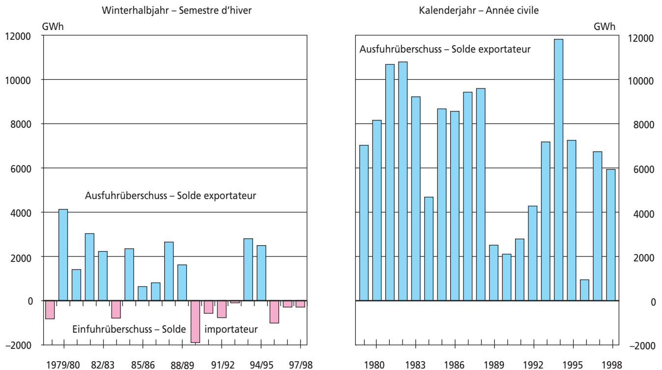
Fig. 19 Ausfuhr- und Einfuhrüberschuss – Solde exportateur et importateur
