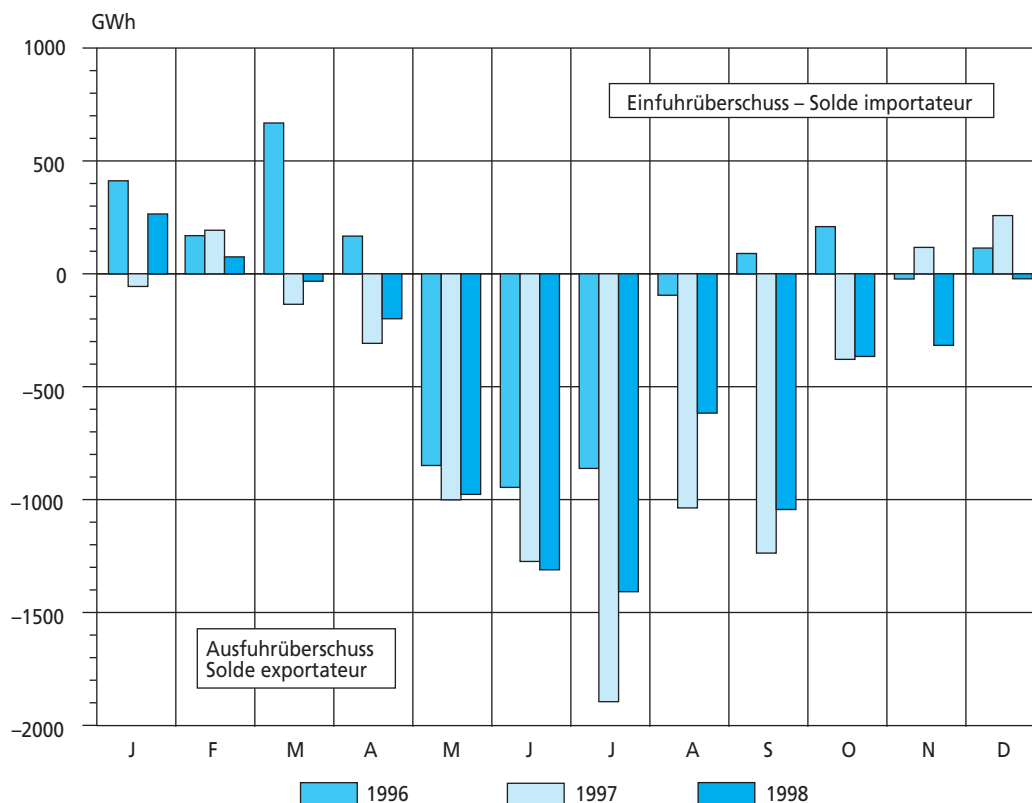
Figur 20 Einfuhr-/Ausfuhrüberschuss (Monatswerte) – Solde importateur/exportateur (chiffres mensuels)
