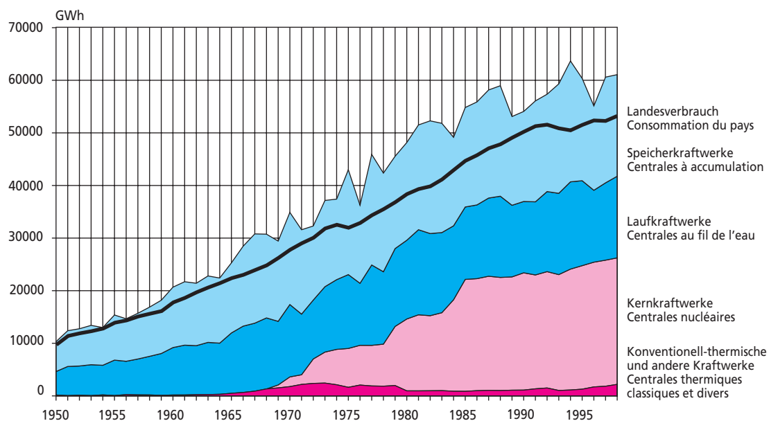
Fig. 9 Evolution des différentes catégories de production depuis 1950
