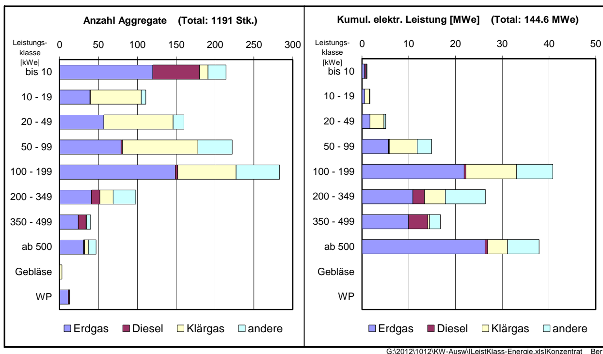
Bild 6.1f Ende 2011 in Betrieb stehende Klein-WKK-Aggregate, geordnet nach Leistungsklassen und nach Energieträgern
