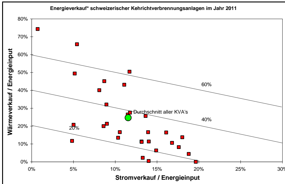
Bild 7.1d Energieverkaufs-Benchmark schweizerischer KVA (Jahr 2011)
