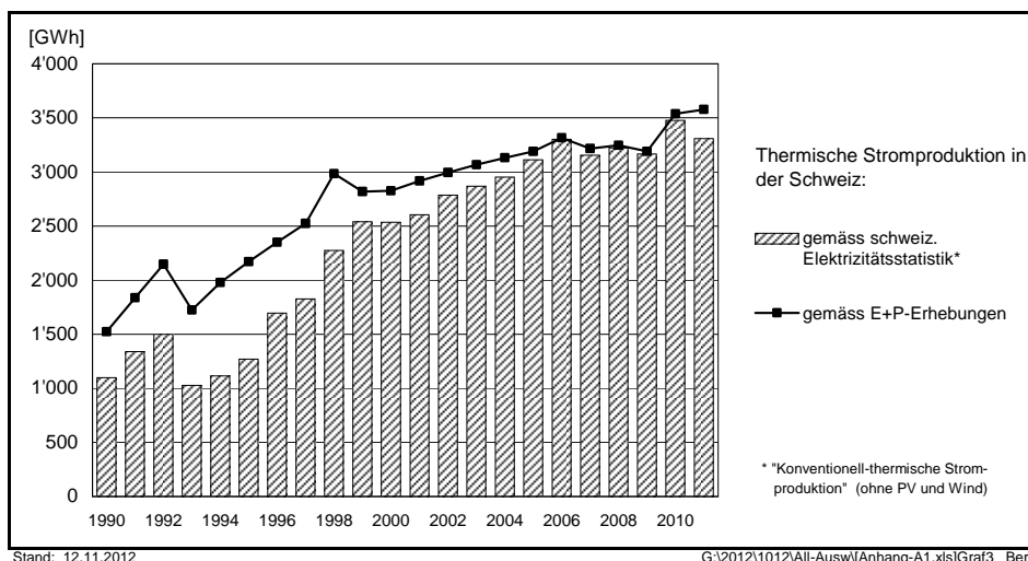
Bild 3.2b Thermische Stromproduktion der Jahre 1990 bis 2011: Vergleich der offiziellen schweizerischen Elektrizitätsstatistik mit den vorliegenden Erhebungsergebnissen
