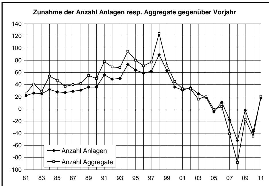
Bild 6.1a Jährliche Zunahme des Klein-WKK-Bestandes
