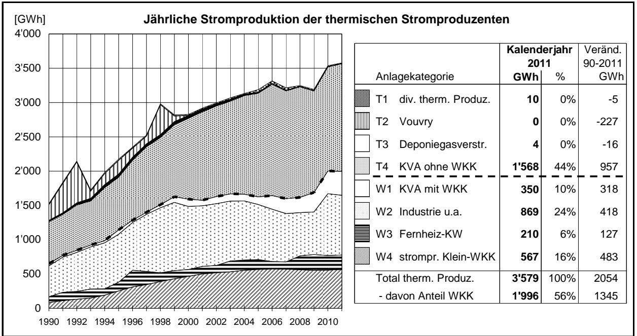
Bild 3.2a Thermische Stromproduktion der Jahre 1990 bis 2011
