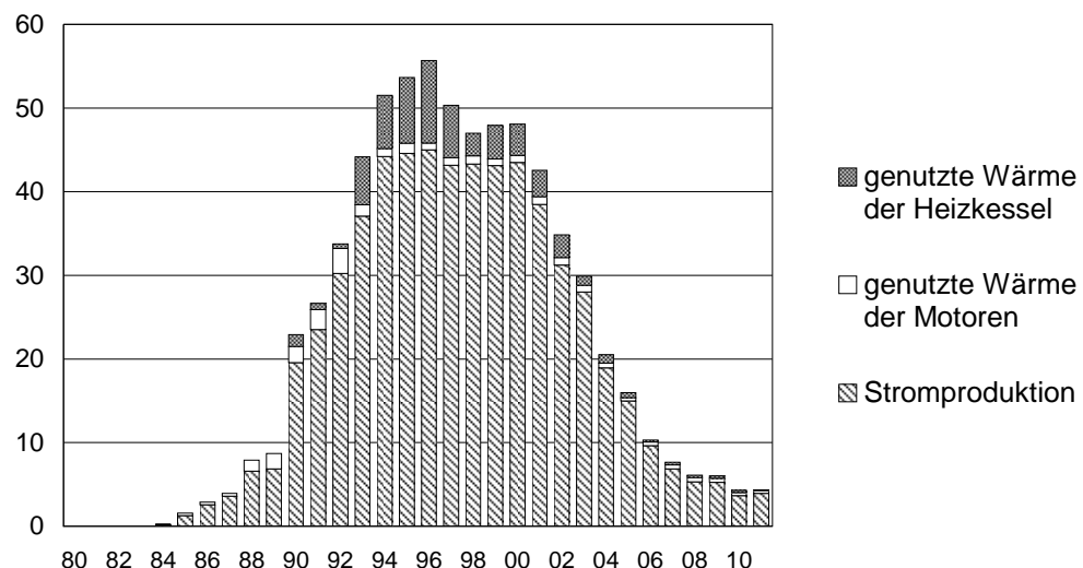
Energienutzung [GWh/a]
