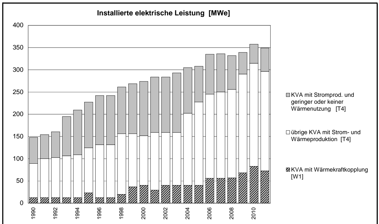
Bild 7.1a Entwicklung der installierten elektrischen Leistung aller Kehrlichtverbrennungsanlagen in der Schweiz (siehe Anhang E.1a)
