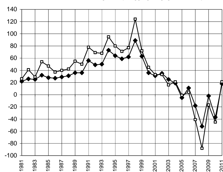
Zunahme der Anzahl Anlagen resp. Aggregate gegenüber Vorjahr
