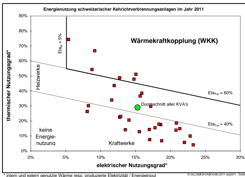
Bild 2.3 Jahresnutzungsgrade der schweizerischen Kehrrechtverbrennungsanlagen im Jahr 2011
