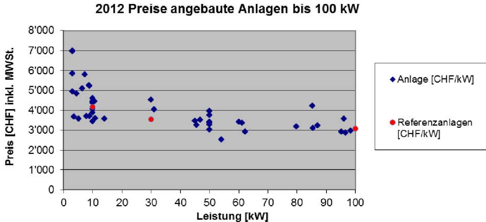
Fig. 6: Bereinigte Daten inkl. den abgeleiteten Kosten für angebaute Referenzanlagen 2012 bis 100 kW
