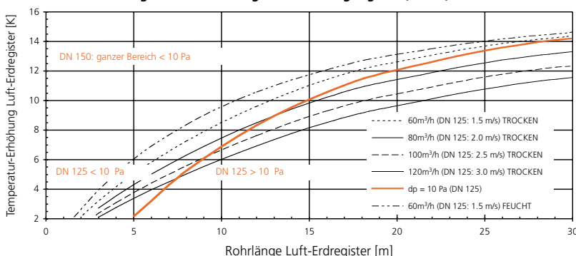
Aussenluft-Erwärmung durch Luft-Erdregister im Auslegungsfall ( -10^\circ\text{C} )
