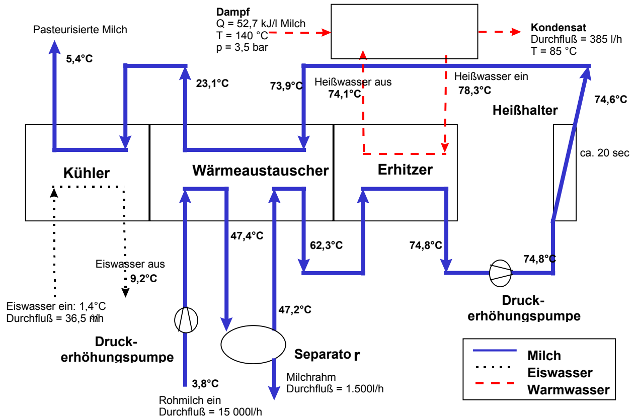
Bild 4.11 Ablaufschema Milcherhitzer 1
