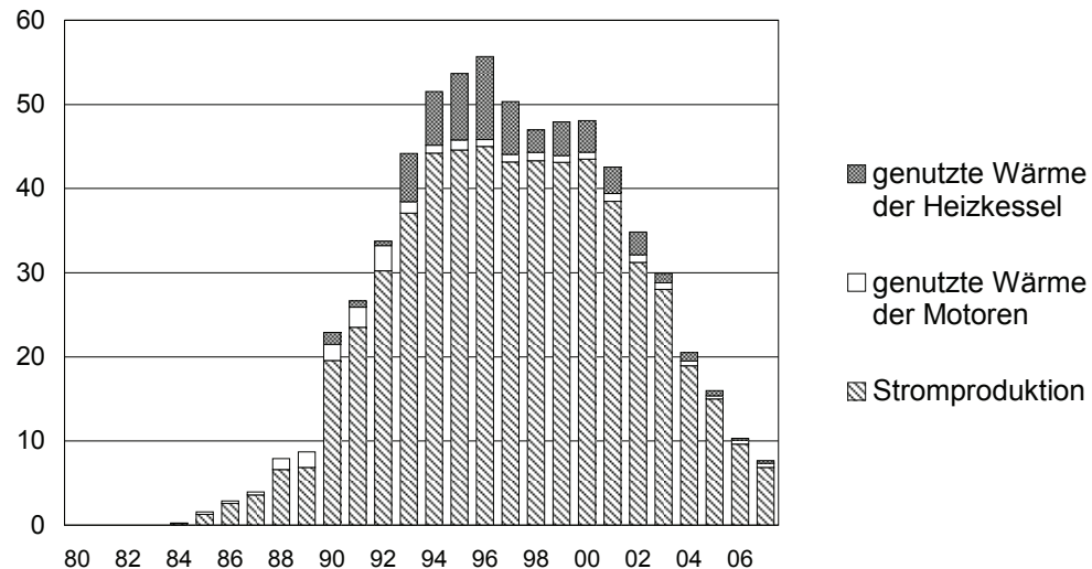
Energienutzung [GWh/a]
