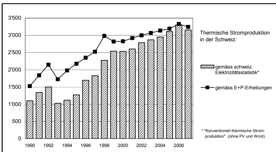
Bild 3.2b Thermische Stromproduktion der Jahre 1990 bis 2007: Vergleich der offiziellen schweizerischen Elektrizitätsstatistik mit den vorliegenden Erhebungsergebnissen
