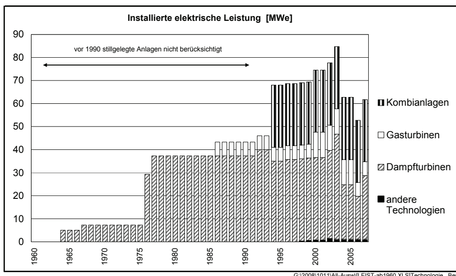
Bild 5.3a Gross-WKK-Anlagen in Fernheizkraftwerken aufgeteilt nach Technologien (siehe Anhang Ce)
