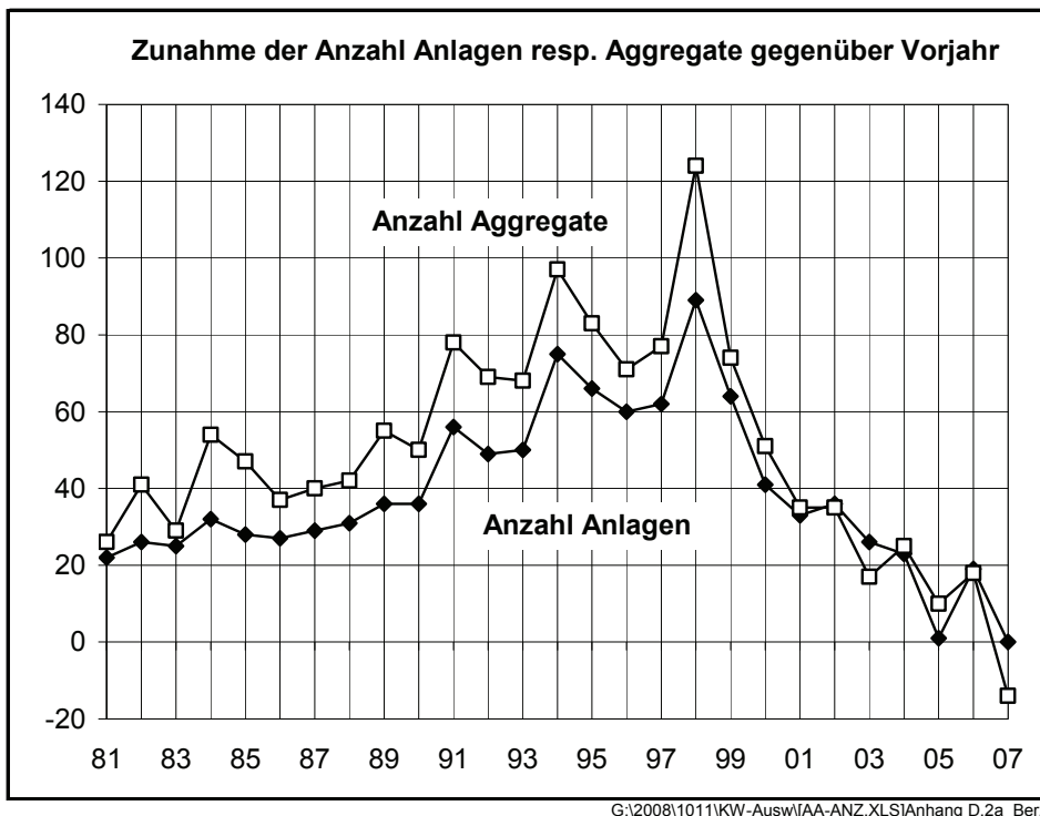
Bild 6.1a Jährliche Zunahme des Klein-WKK-Bestandes (siehe Anhang D.2a)
