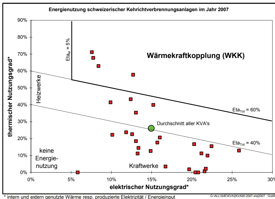
Bild 2.3 Jahresnutzungsgrade der schweizerischen Kehrichtverbrennungsanlagen im Jahr 2007
