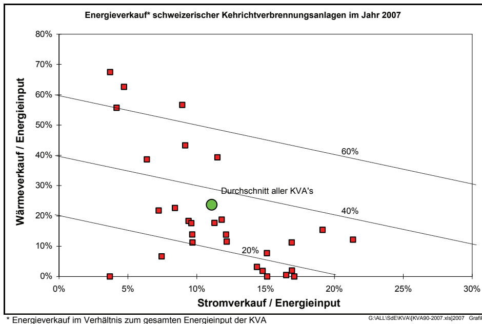
Bild 7.1d Energieverkaufs-Benchmark schweizerischer KVA's (Jahr 2007)
