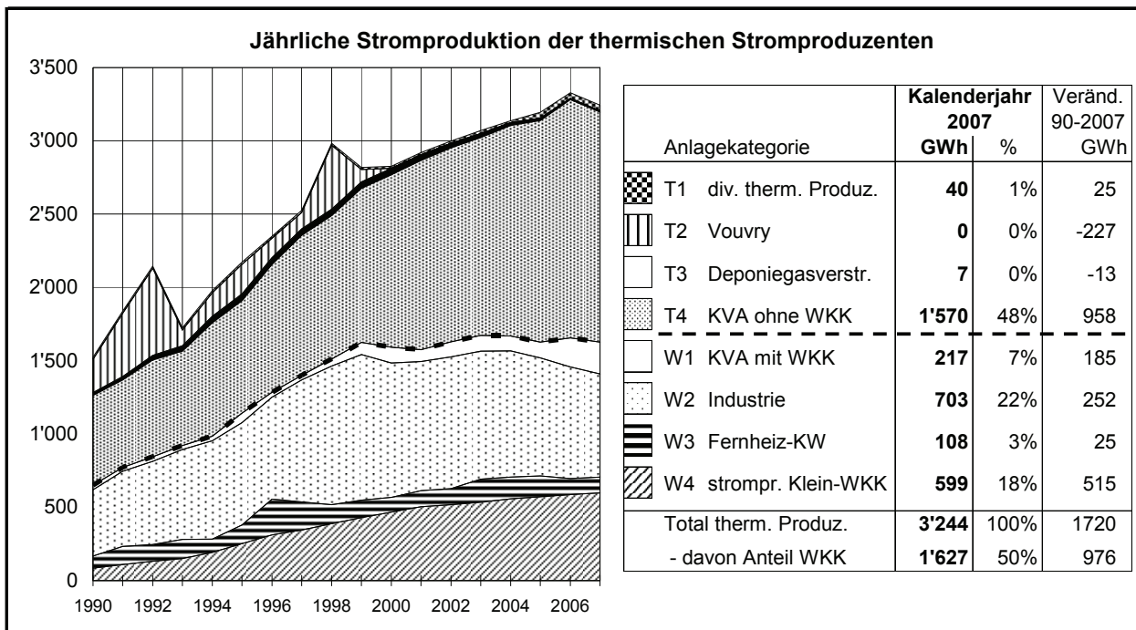
Bild 3.2a Thermische Stromproduktion der Jahre 1990 bis 2007
