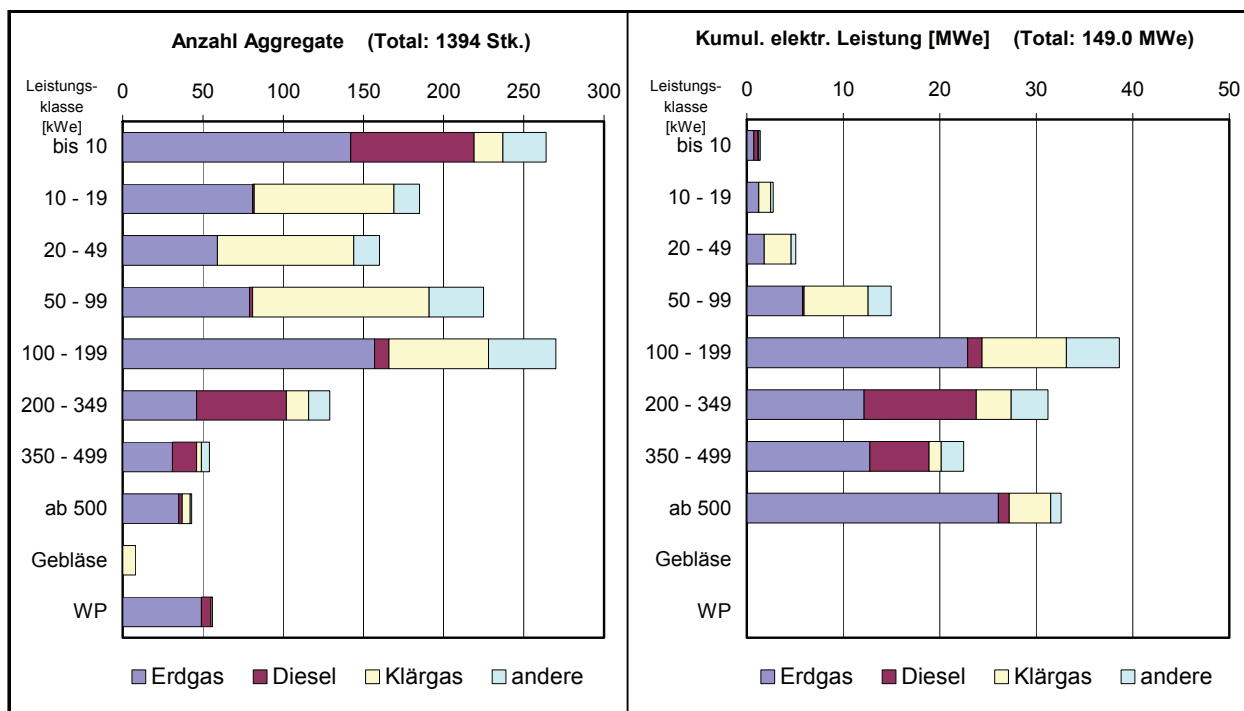
Bild 6.1f Ende 2007 in Betrieb stehende Klein-WKK-Aggregate, geordnet nach Leistungsklassen und nach Energieträgern
