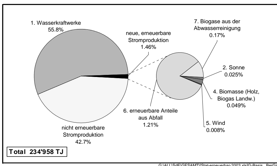
Bild 1.6 Gesamte schweizerische Elektrizitätsproduktion 2003 (Gliederung nach Technologien gemäss Bild 1.1)
