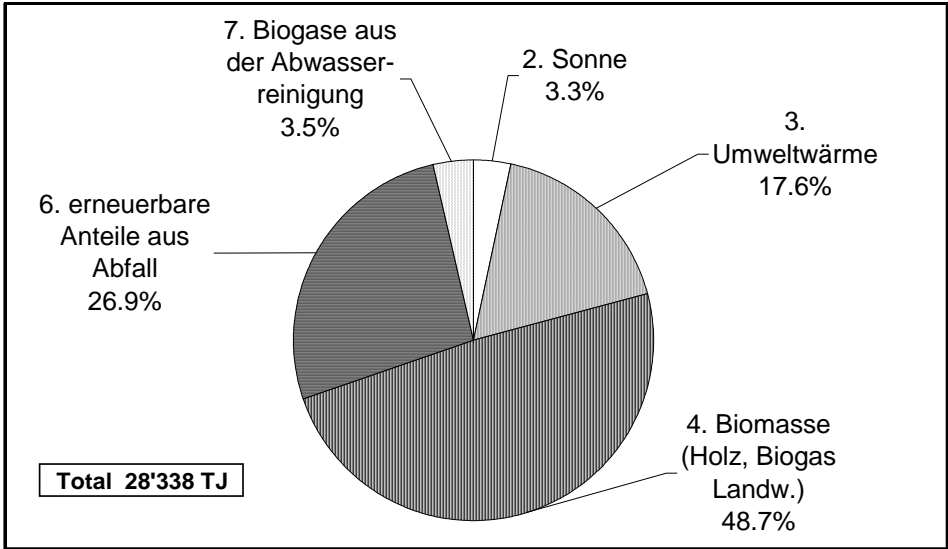
Bild 1.8 Genutzte erneuerbare Wärme 2003 ("Nutzenergie" am Speicheraustritt in der Heizzentrale; Gliederung nach Technologien gemäss Bild 1.1)
