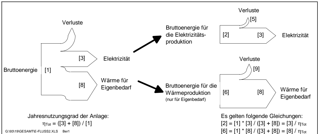
Bild 2.7 Ermittlung der Bruttoenergien für die Elektrizitäts- und für die Eigenbedarfswärmeherstellung (Beispiel einer Anlage ohne Fernwärmeherstellung)
