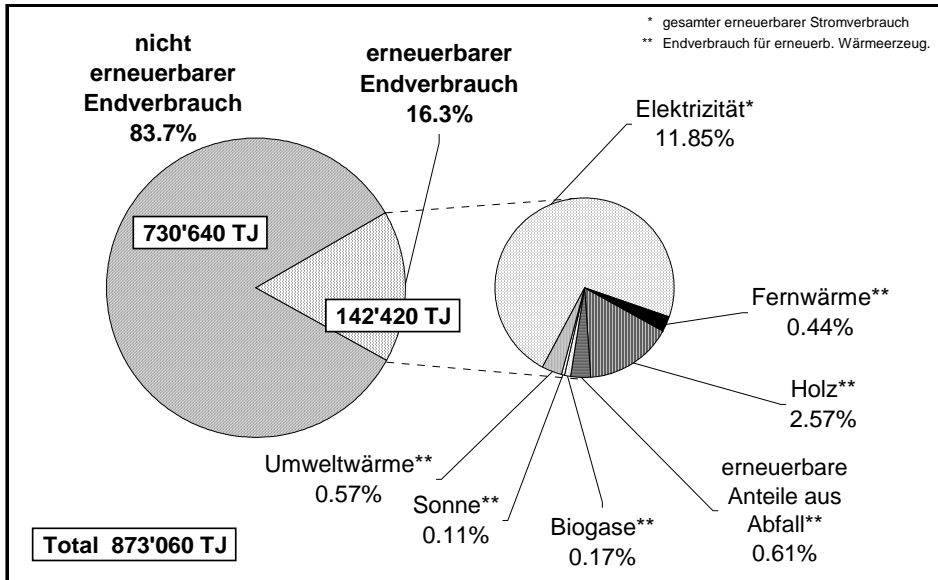
Bild 1.4 Gesamter schweizerische Endenergieverbrauch 2003 mit den erneuerbaren Anteilen (Gliederung nach Energieträgern)
