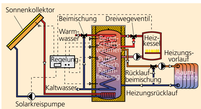
Solares Heizsystem
