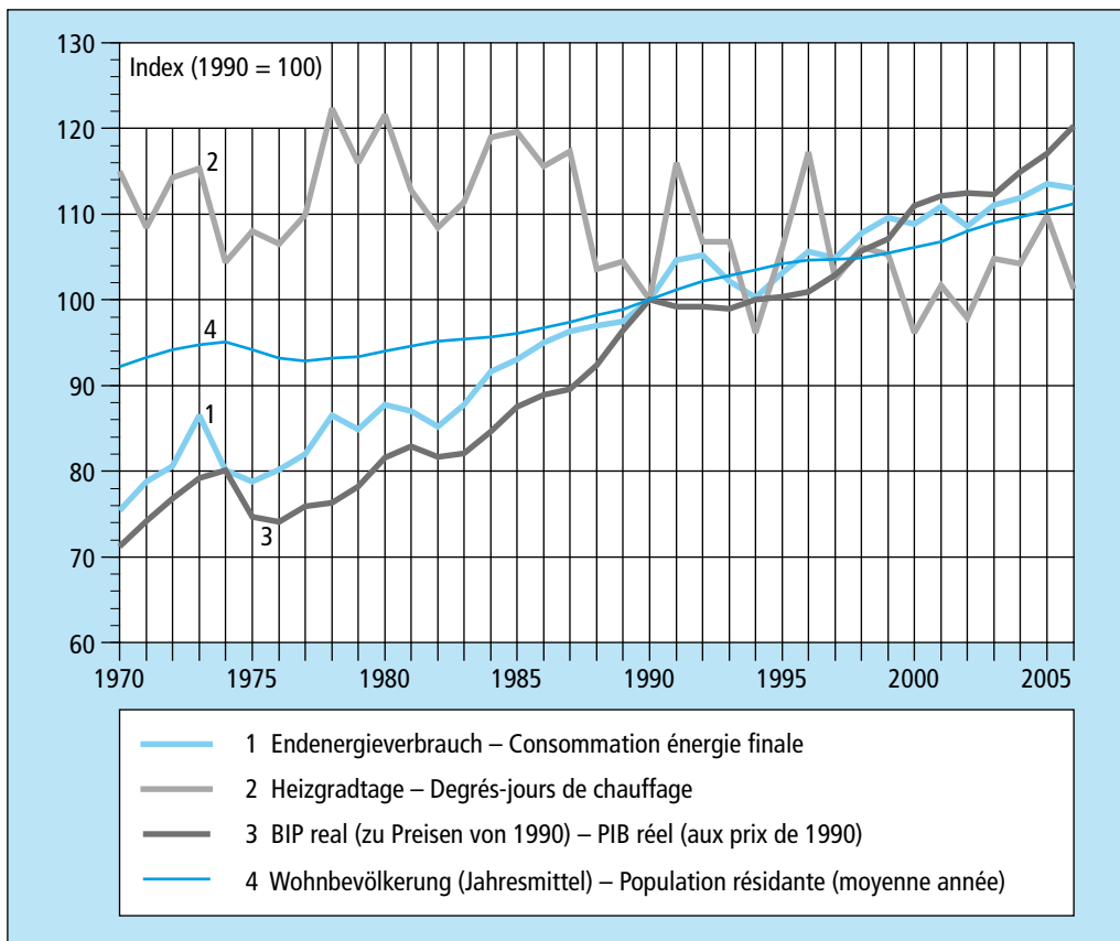
Fig. 14 Entwicklung energierelevanter Grössen im Vergleich zum Endverbrauch
