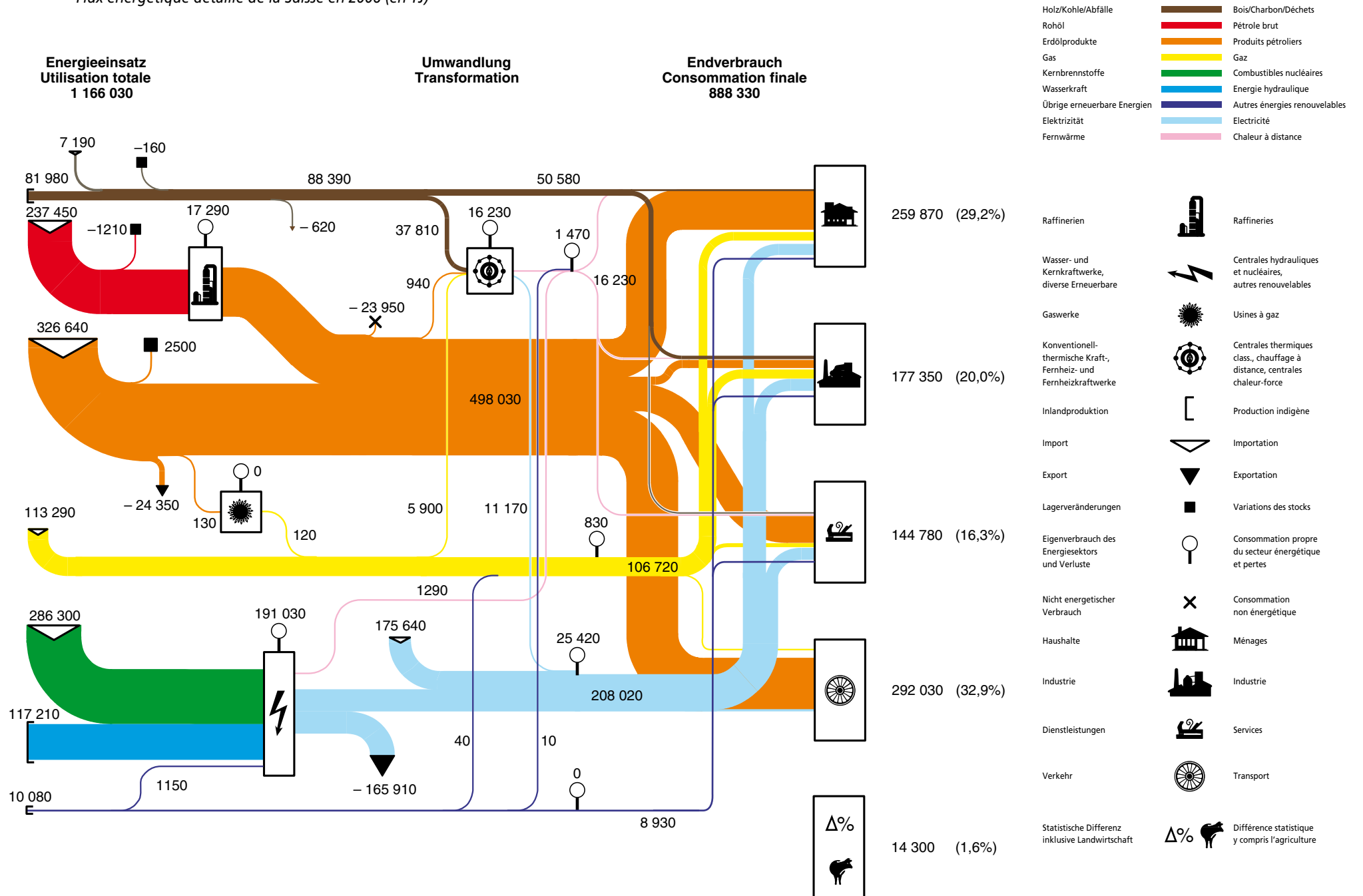
Fig. 5 Detailliertes Energieflussdiagramm der Schweiz 2006 (in TJ) Flux énergétique détaillé de la Suisse en 2006 (en TJ)
