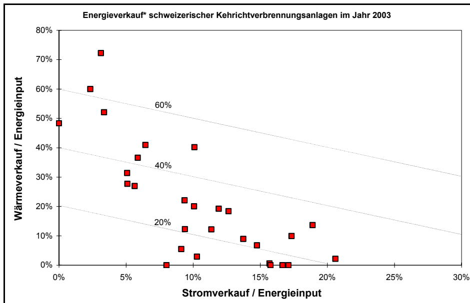
Bild 7.1d Energieverkaufs-Benchmark schweizerischer KVA's (Jahr 2003)
