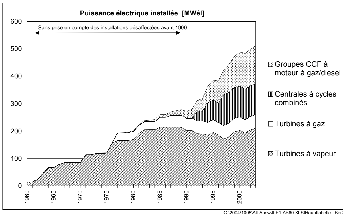
Figure 1.2 Evolution de la puissance électrique des installations à CCF selon leur type
