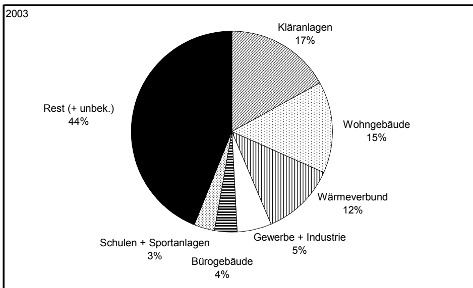
Bild 6.2d Neuinstallierte Klein-WKK-Leistung nach Einsatzgebieten (Jahr 2003)
