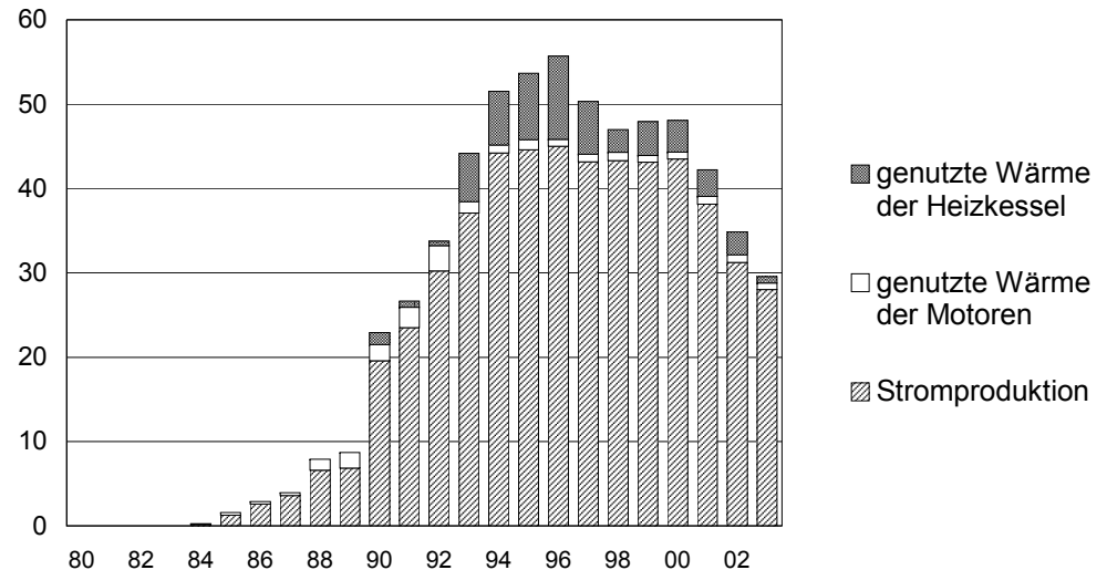
Energienutzung [GWh/a]
