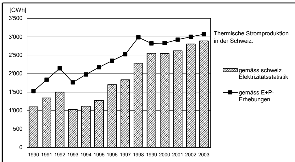
Bild 3.2b Thermische Stromproduktion der Jahre 1990 bis 2003: Vergleich der offiziellen schweizerischen Elektrizitätsstatistik mit den vorliegenden Erhebungsergebnissen
