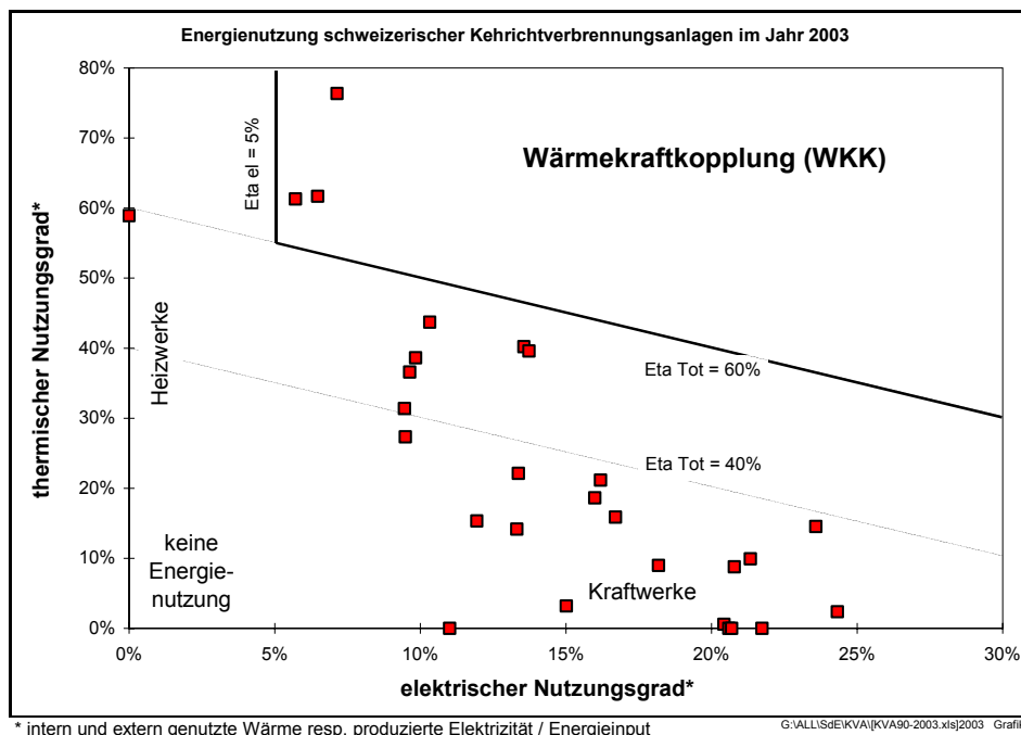
Bild 2.3 Jahresnutzungsgrade der schweizerischen Kehrichtverbrennungsanlagen im Jahr 2003
