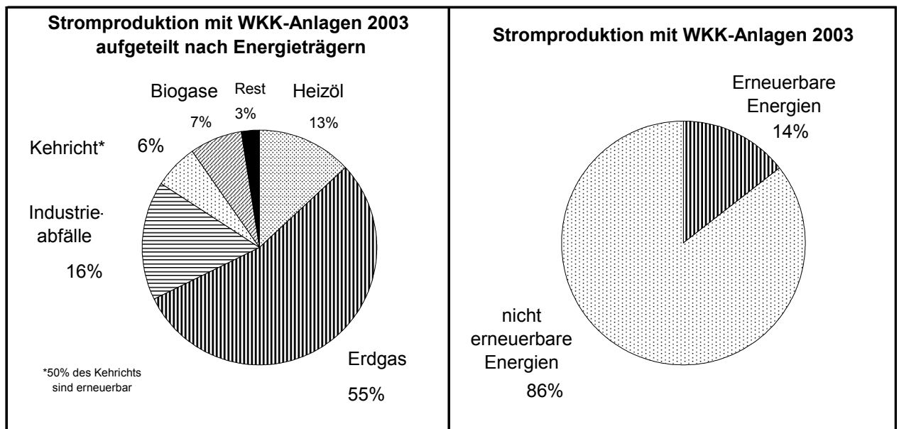
Bild 4.2 Aufteilung der WKK-Stromproduktion 2003 nach Energieträgern
