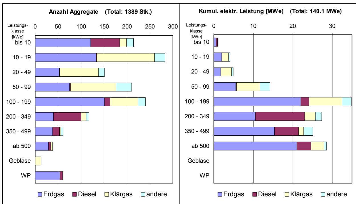
Bild 6.1f Ende 2003 in Betrieb stehende Klein-WKK-Aggregate, geordnet nach Leistungsklassen und nach Energieträgern (siehe Anhang D.2g)
