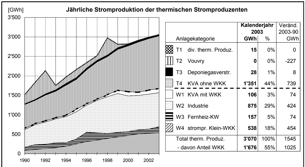
Bild 3.2a Thermische Stromproduktion der Jahre 1990 bis 2003
