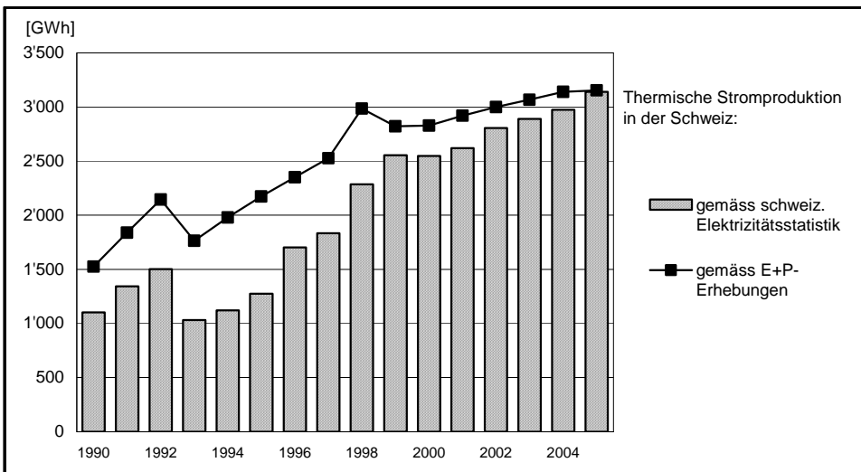
Bild 3.2b Thermische Stromproduktion der Jahre 1990 bis 2005: Vergleich der offiziellen schweizerischen Elektrizitätsstatistik mit den vorliegenden Erhebungsergebnissen
