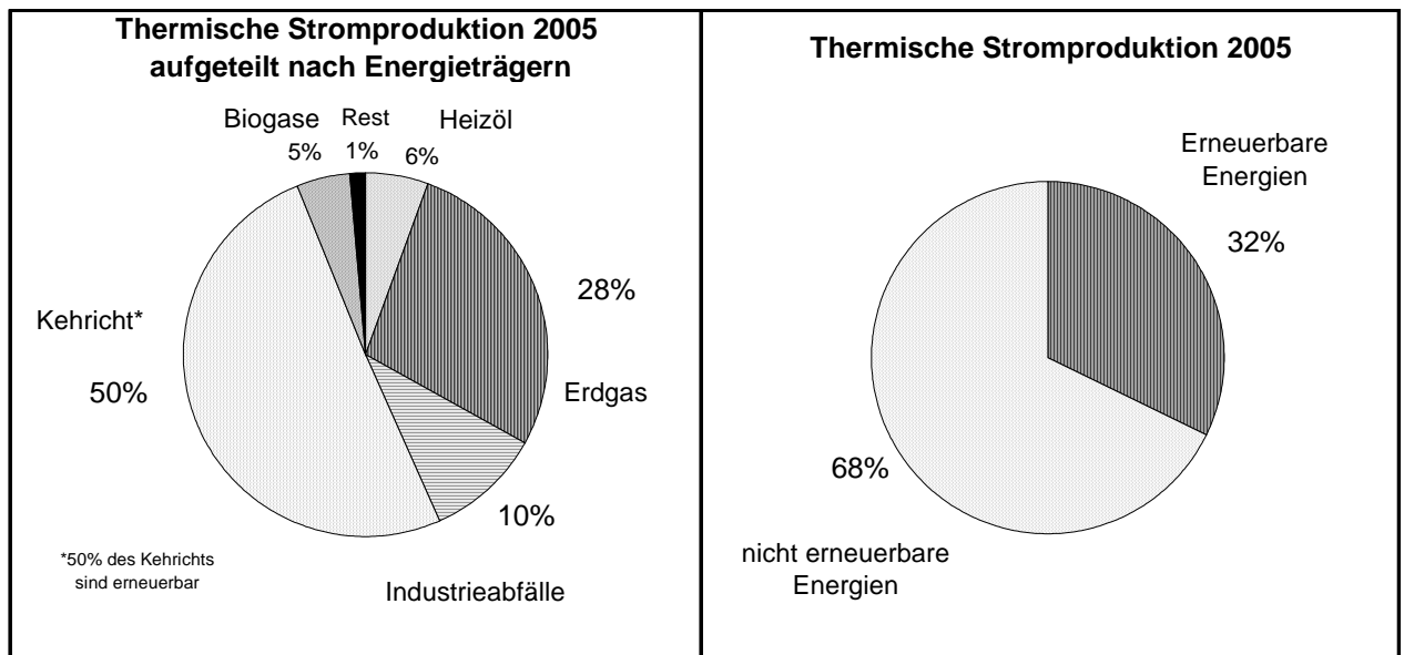
Bild 3.3 Thermische Stromproduktion 2005 aufgeteilt nach Energieträgern. Der relative hohe Anteil erneuerbarer Energien von 32 % an der thermischen Stromproduktion liegt darin begründet, dass rund 50 % des verbrannten Kehrichts erneuerbaren Ursprungs ist. (siehe Anhang A.2)
