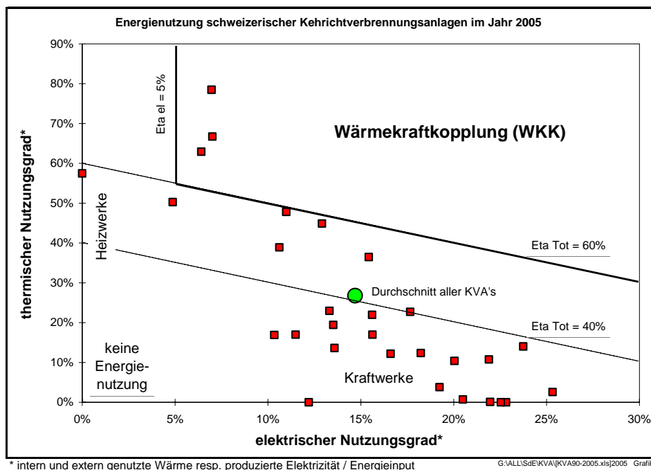
Bild 2.3 Jahresnutzungsgrade der schweizerischen Kehrrechtverbrennungsanlagen im Jahr 2005
