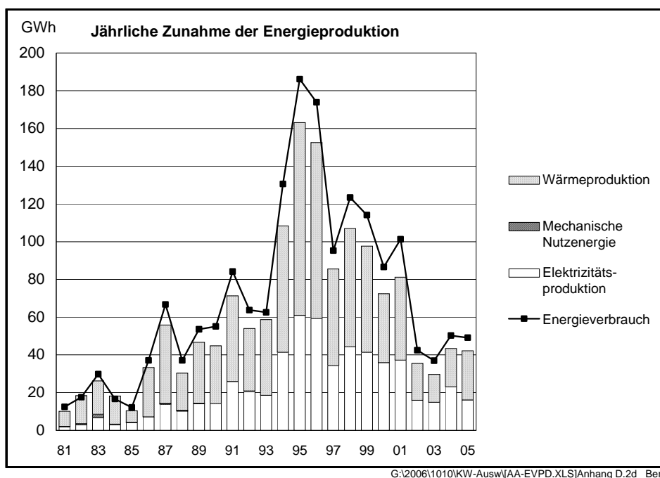
Bild 6.1h Jährliche Zunahmen der Energieproduktion resp. des Energieverbrauchs der Klein-WKK-Anlagen (siehe Anhang D.2d)
