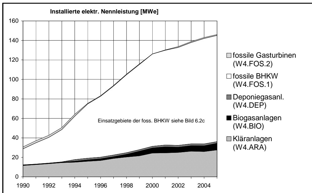
Bild 6.2b Entwicklung der elektrischen Nennleistungen der Klein-WKK-Anlagen nach Anlagekategorien
