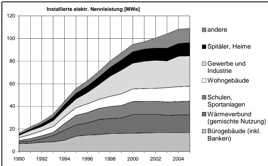
Bild 6.2c Entwicklung der elektrischen Nennleistungen fossiler BHKW nach Einsatzgebieten
