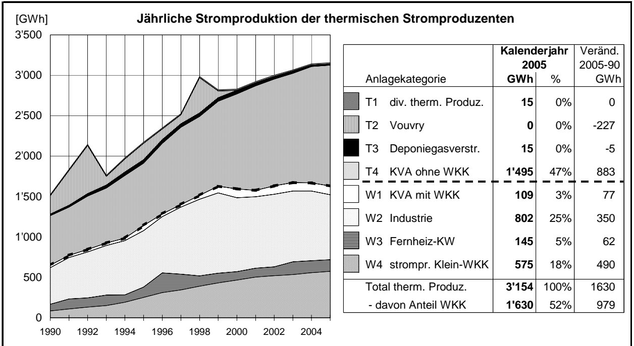
Bild 3.2a Thermische Stromproduktion der Jahre 1990 bis 2005
