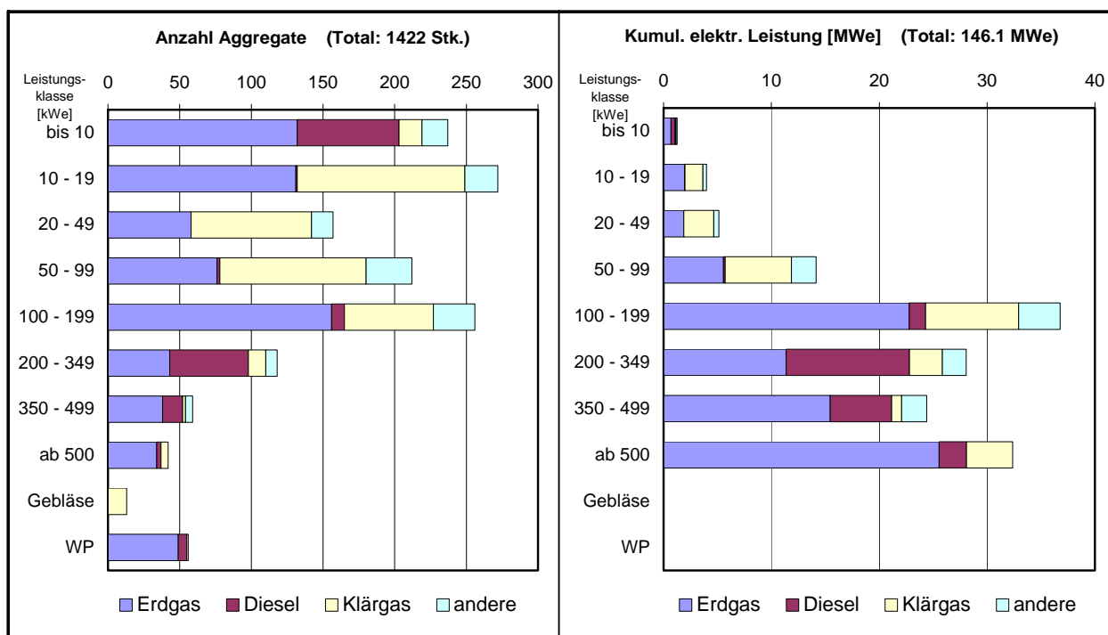
Bild 6.1f Ende 2005 in Betrieb stehende Klein-WKK-Aggregate, geordnet nach Leistungsklassen und nach Energieträgern
