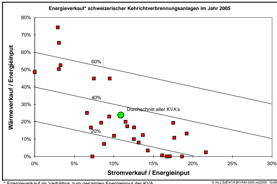
Bild 7.1d Energieverkaufs-Benchmark schweizerischer KVA's (Jahr 2005)
