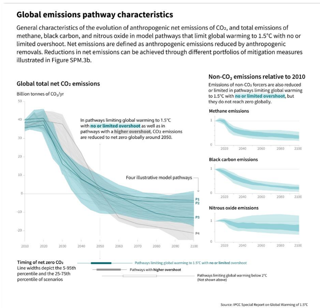
Abbildung 16: Absenkszenarien für Treibhausgase, gemässe IPCC Spezialreport für das 1.5°C-Ziel 99
