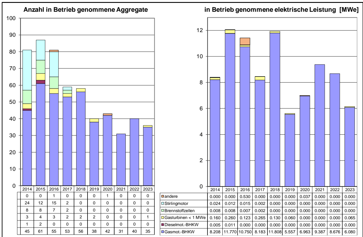
Bild 6.4c In Betrieb genommene Klein-WKK-Aggregate der letzten 10 Jahre
