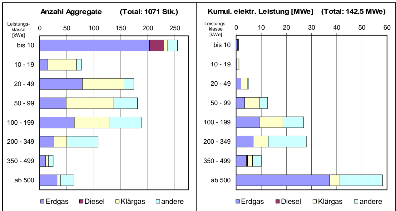
Bild 6.1f Ende 2023 in Betrieb stehende Klein-WKK-Aggregate, geordnet nach Leistungsklassen und nach Energieträgern
