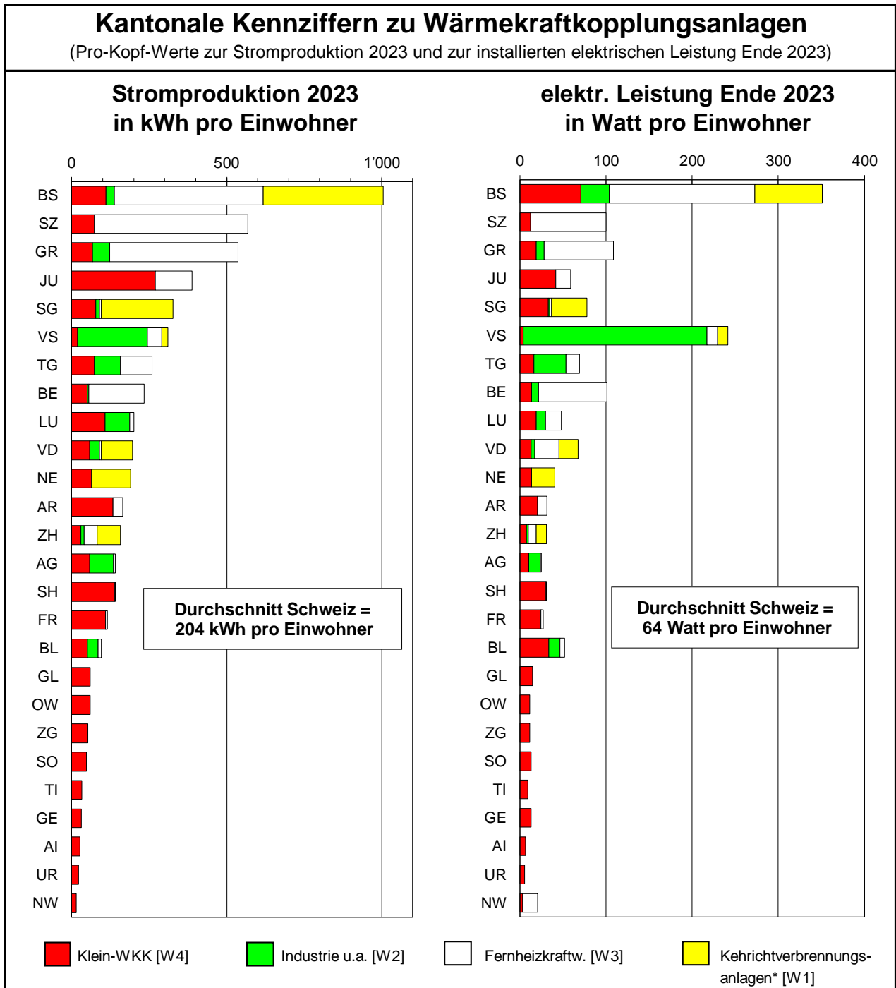
Bild 4.3 Kantonale Pro-Kopf-Werte aller WKK-Anlagen
