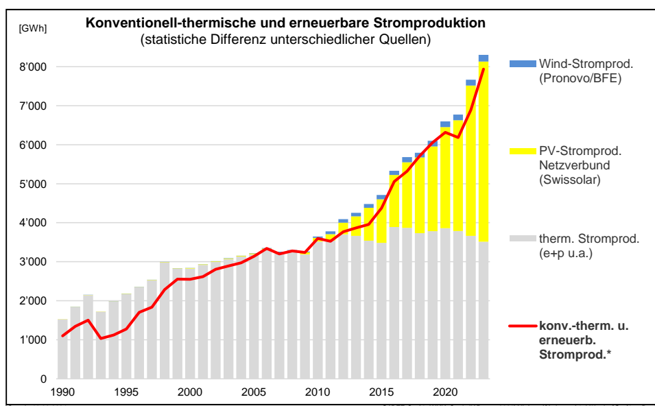
Bild 3.2b Stromproduktion „thermisch und andere“: Vergleich der schweiz. Elektrizitätsstatistik (rot) mit den Erhebungen von e+p, Swissolar und Pronovo/BFE (Balken)
