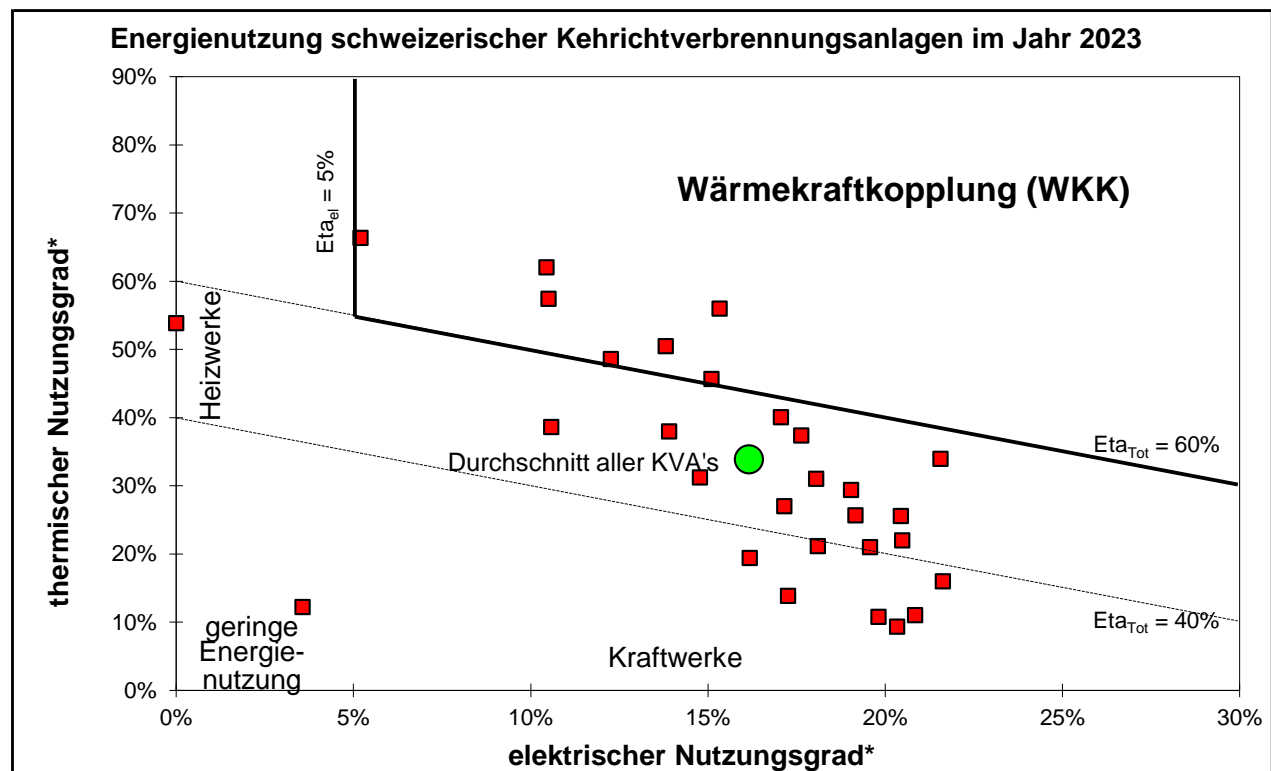
Bild 2.3 Jahresnutzungsgrade der schweizerischen Kehrichtverbrennungsanlagen im Jahr 2023
