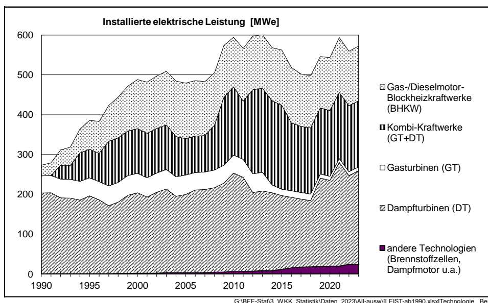
Bild 4.1c Elektrische Nennleistungen der WKK-Anlagen aufgeteilt nach Technologien (siehe Anhang B.1b)
