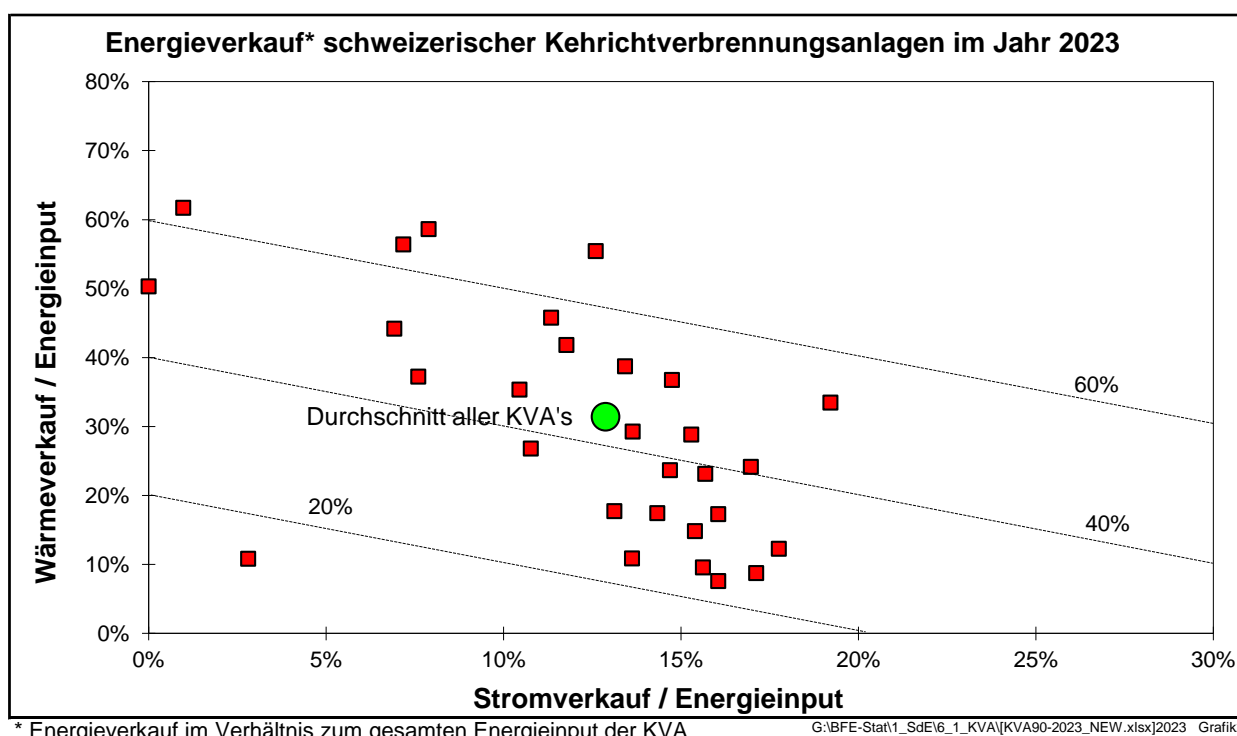
Bild 7.1d Energieverkaufs-Benchmark schweizerischer KVA (Jahr 2023)
