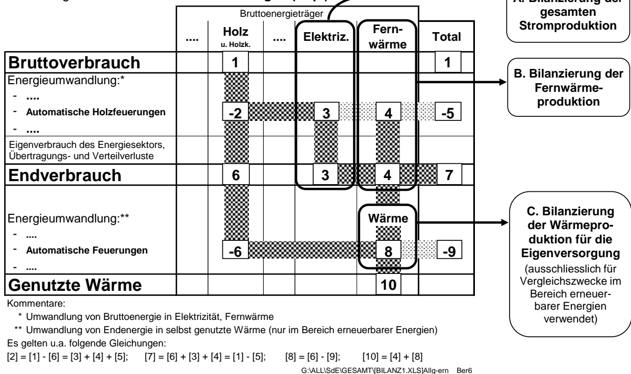
Bild 2.6 Schematische Darstellung der verwendeten Bilanzierung erneuerbarer Energien (Bsp. automatische Holzfeuerungen)
