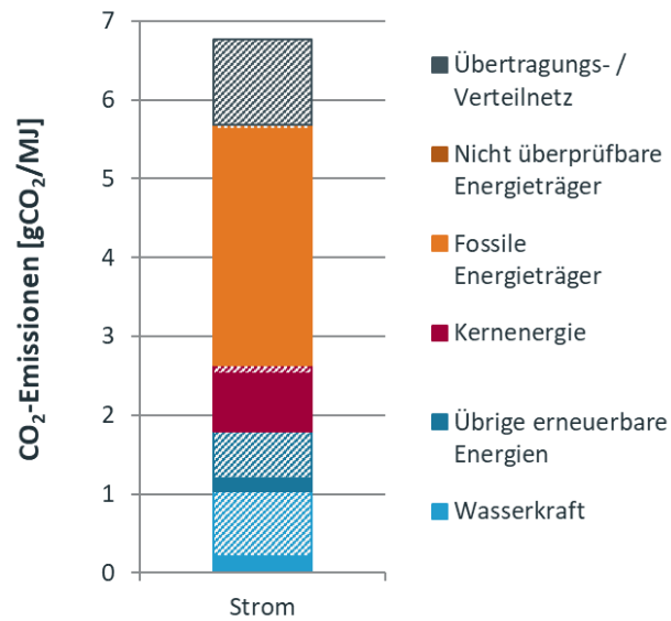
Fig. A.2 Beiträge der wichtigsten Stromqualitäten und des Übertragungs- und Verteilnetzes zu den fossilen CO 2 -Emissionen des HKN-Lieferantenstrommix Schweiz 2022. Die Beiträge der Infrastruktur werden für jeden Prozess separat als schraffierte Flächen dargestellt.
