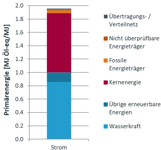
Fig. A.1 Beiträge der wichtigsten Stromqualitäten und des Übertragungs- und Verteilnetzes zur Primärenergie des HKN-Lieferantenstrommix Schweiz 2022. Die Beiträge der Infrastruktur werden für jeden Prozess separat als schraffierte Flächen dargestellt.
