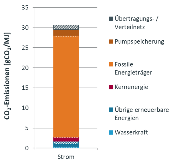
Fig. 4.5 Beiträge der wichtigsten Prozesse zu den fossilen CO 2 -Emissionen von Strom (Verbraucherstrommix Schweiz 2020-2022). Die Beiträge der Infrastruktur werden für jeden Prozess separat als schraffierte Flächen dargestellt.
