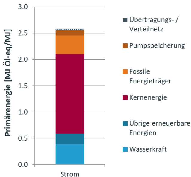
Fig. 4.4 Beiträge der wichtigsten Prozesse zur Primärenergie von Strom (Verbraucherstrommix Schweiz 2020-2022). Die Beiträge der Infrastruktur werden für jeden Prozess separat als schraffierte Flächen dargestellt.
