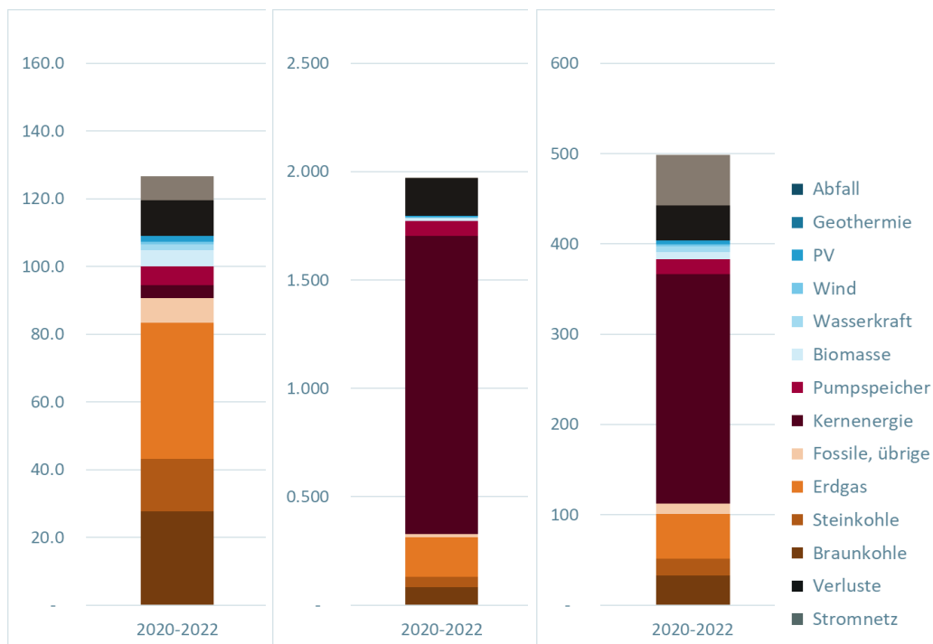
Fig. 4.3 Umweltkennwerte (links: Treibhausgasemissionen (g CO 2 -eq), Mitte: Primärenergiebedarf nicht erneuerbar (MJ Öl-eq), rechts: Gesamtweltbelastung (UBP) gemäss Ökofaktoren 2021 der Methode der ökologischen Knappheit) von 1 kWh des Schweizer Verbraucherstrommix basierend auf Produktion und kommerziellem Handel 2020-2022.
