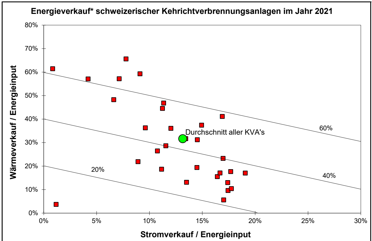
Bild 7.1d Energieverkaufs-Benchmark schweizerischer KVA (Jahr 2021)
