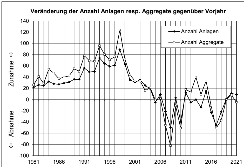
Bild 6.1a Jährliche Veränderung des Klein-WKK-Bestandes (siehe Anhang D.2a)
