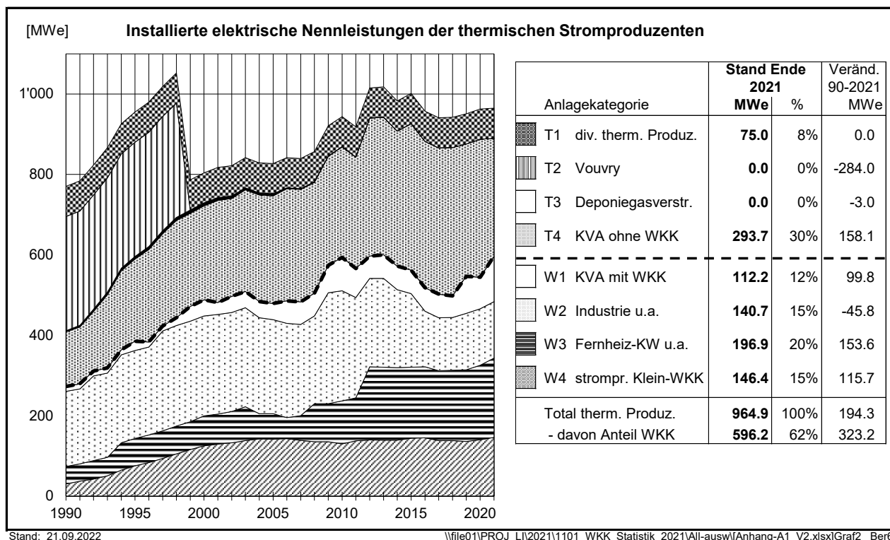
Bild 3.1b Entwicklung der installierten elektrischen Nennleistungen
