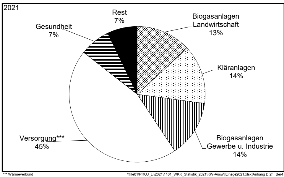
Bild 6.2d Neuinstallierte Klein-WKK-Leistung nach Einsatzgebieten (Jahr 2021)
