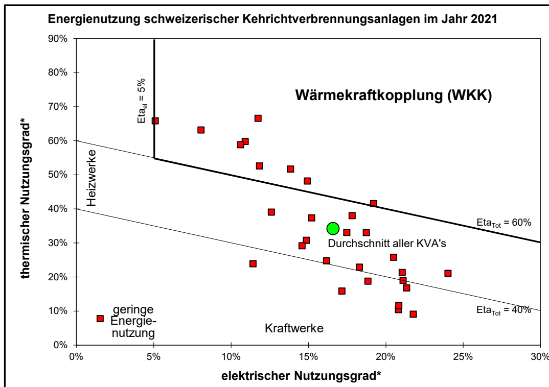
Bild 2.3 Jahresnutzungsgrade der schweizerischen Kehrichtverbrennungsanlagen im Jahr 2021
