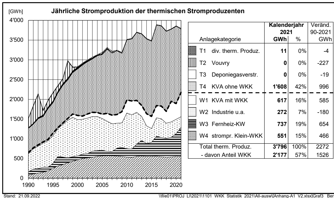
Bild 3.2a Thermische Stromproduktion der Jahre 1990 bis 2021
