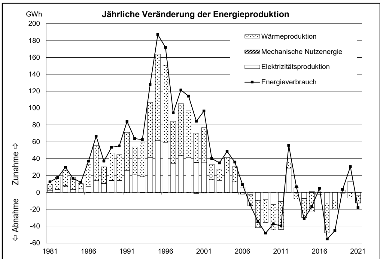
Bild 6.1h Jährliche Veränderung der Energieproduktion und des Energieverbrauchs der Klein-WKK-Anlagen (siehe Anhang D.2d)
