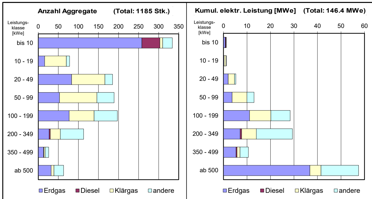
Bild 6.1f Ende 2021 in Betrieb stehende Klein-WKK-Aggregate, geordnet nach Leistungsklassen und nach Energieträgern
