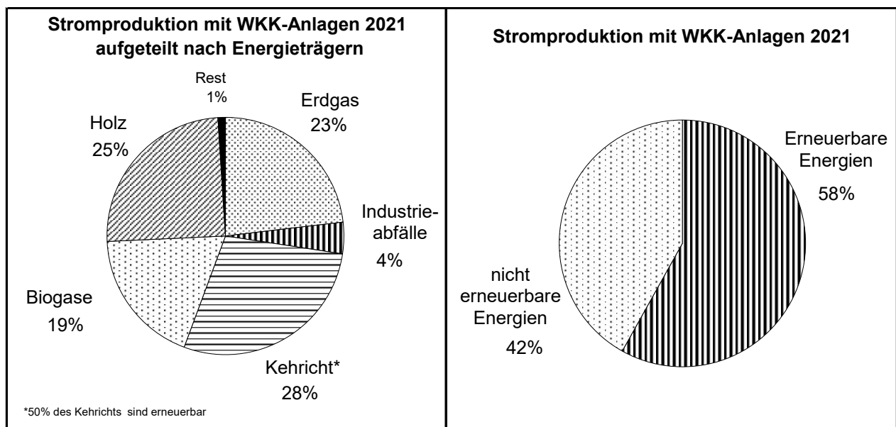
Bild 4.2 Aufteilung der WKK-Stromproduktion 2021 nach Energieträgern
