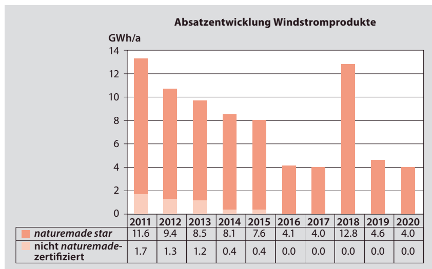
Abbildung 17: Verkaufte Strommengen aus Windstromprodukten, differenziert nach der Qualität, ohne Windanteil aus Mixprodukten.
