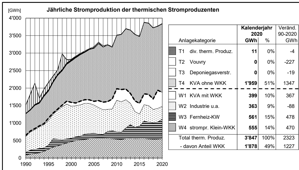
Bild 3.2a Thermische Stromproduktion der Jahre 1990 bis 2020
