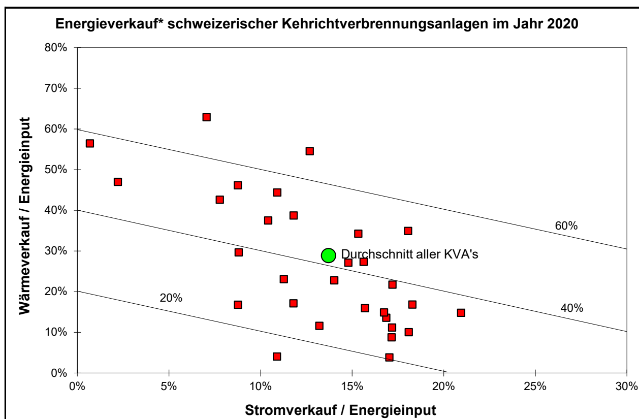
Bild 7.1d Energieverkaufs-Benchmark schweizerischer KVA (Jahr 2020)
