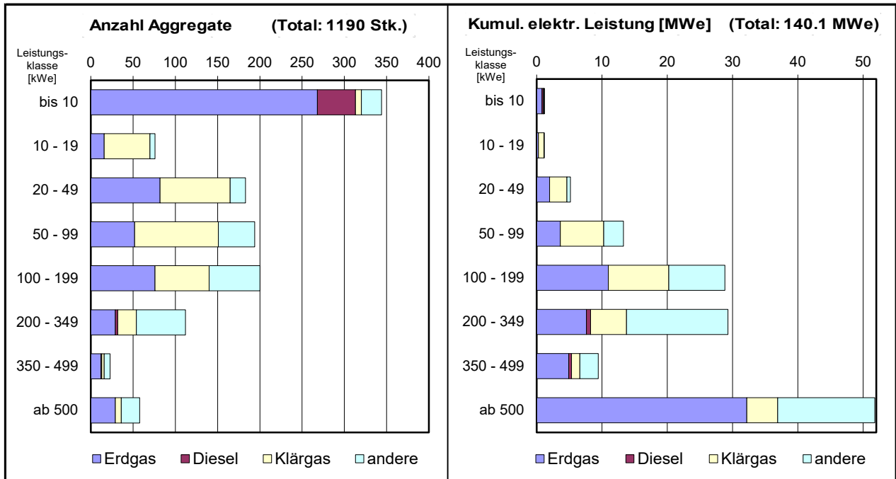
Bild 6.1f Ende 2020 in Betrieb stehende Klein-WKK-Aggregate, geordnet nach Leistungsklassen und nach Energieträgern
