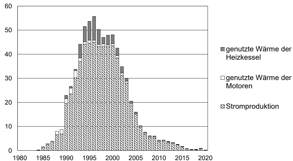
Energienutzung [GWh/a]
