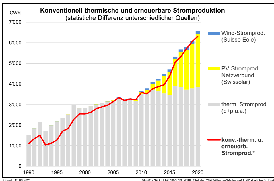
Bild 3.2b Stromproduktion „thermisch und andere“: Vergleich der schweizerischen Elektrizitätsstatistik (rot) mit den Erhebungen von e+p, Swissolar und Suisse Eole (Balken)
