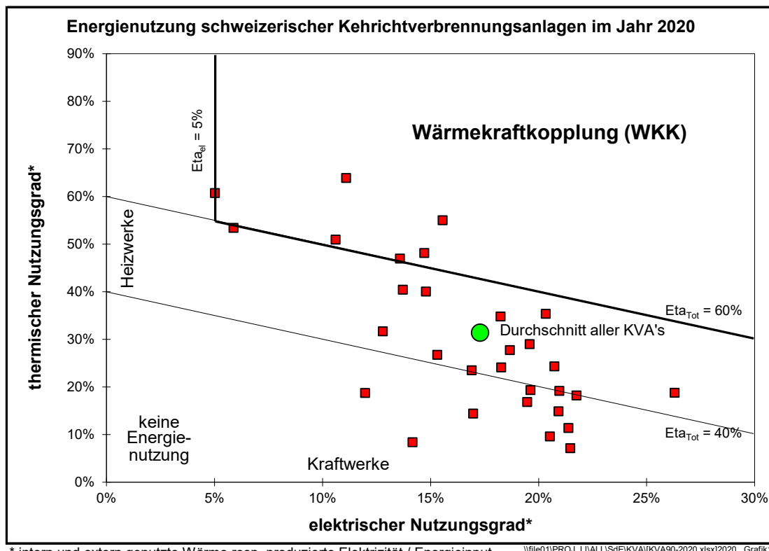
Bild 2.3 Jahresnutzungsgrade der schweizerischen Kehrichtverbrennungsanlagen im Jahr 2020
