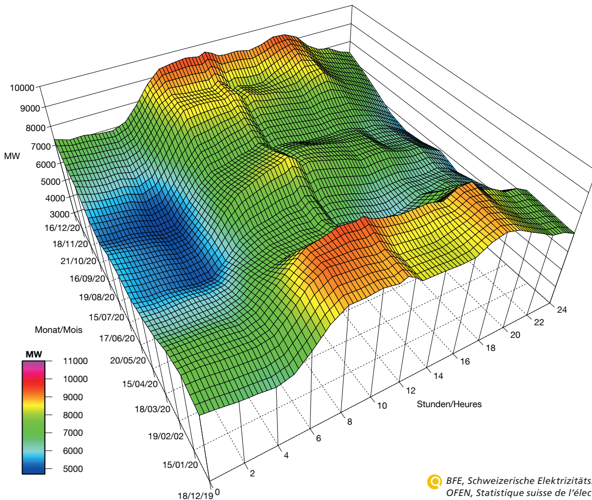
Fig. 18 Belastungswerte 2020 der schweizerischen Elektrizitätswerke Charge horaire et mensuelle des centrales électriques suisses en 2020
