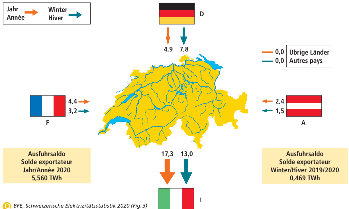
Fig. 3 Einfuhr-/Ausfuhrsaldo 2020 (in TWh), physikalische Werte Solde importateur/exportateur 2020 (en TWh), valeurs physiques
