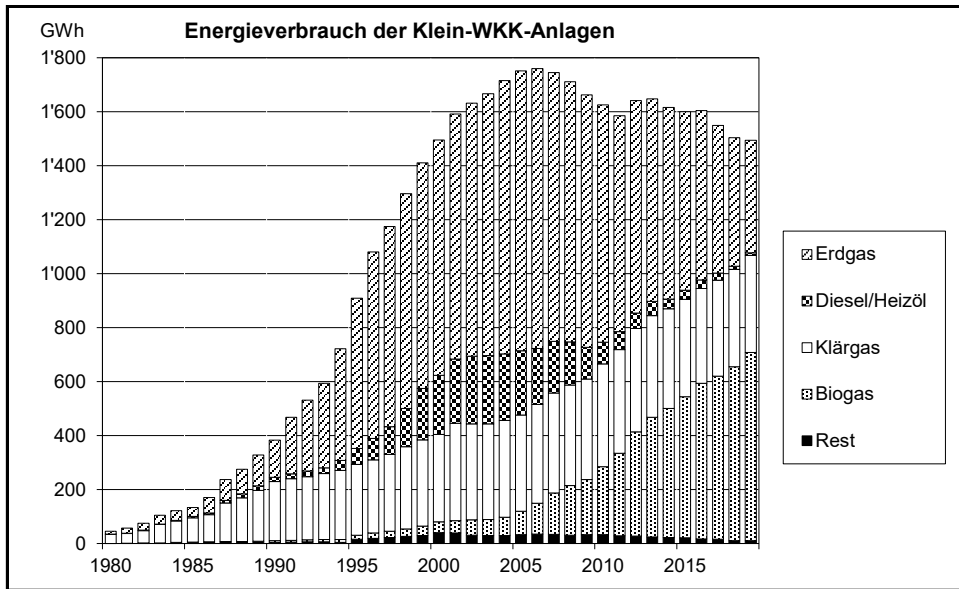
Bild 6.1i Entwicklung des Energieverbrauchs aller schweizerischer Klein-WKK-Anlagen (siehe Anhang D.2e)
