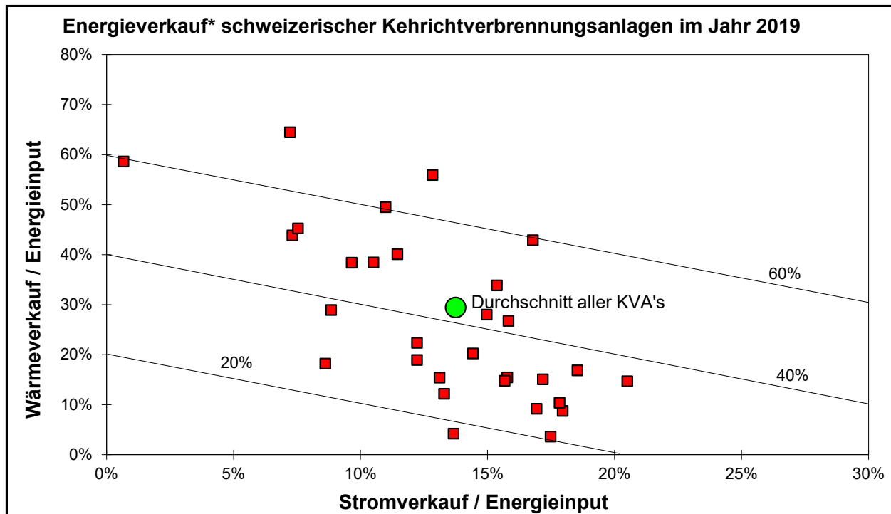
Bild 7.1d Energieverkaufs-Benchmark schweizerischer KVA (Jahr 2019)
