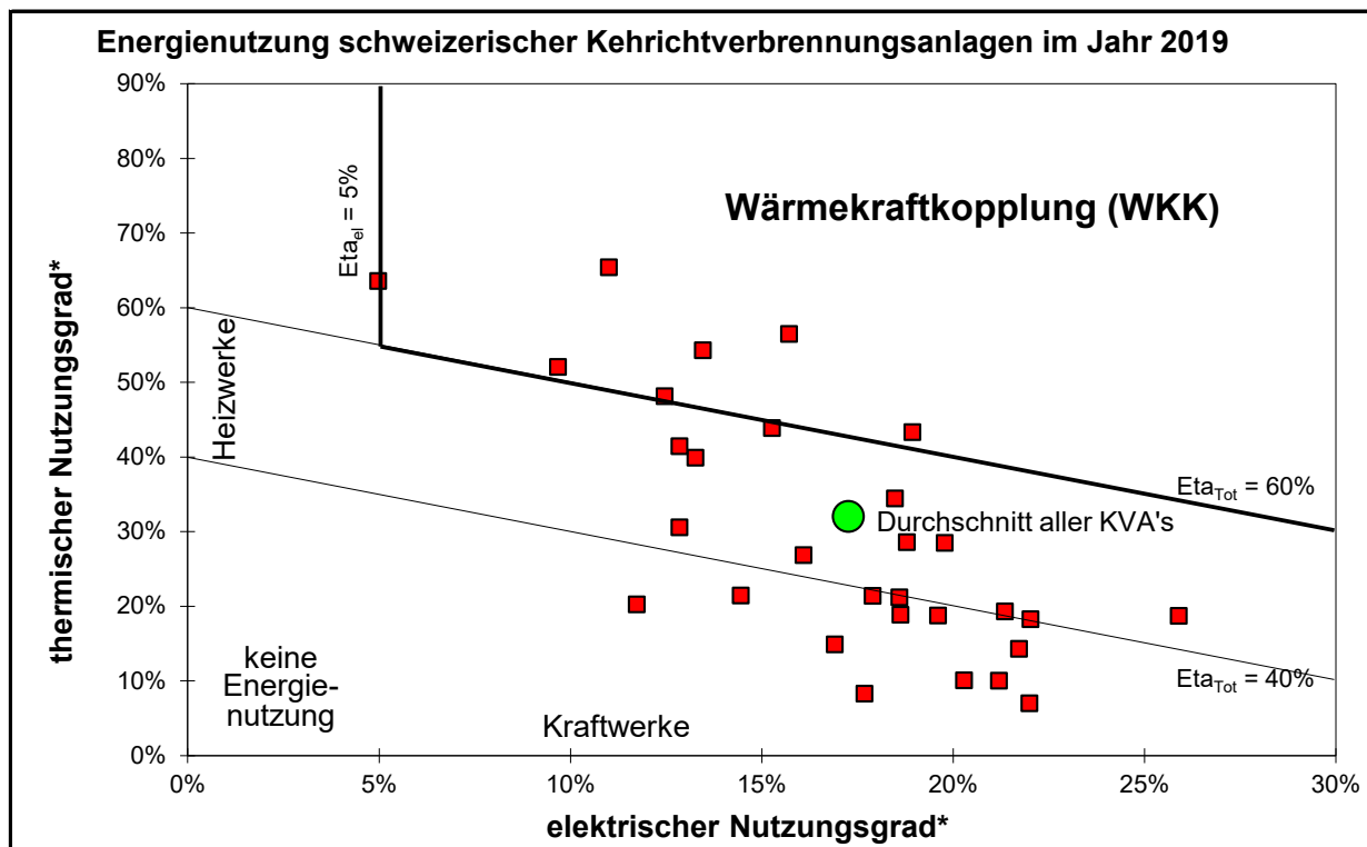
Bild 2.3 Jahresnutzungsgrade der schweizerischen Kehrichtverbrennungsanlagen im Jahr 2019
