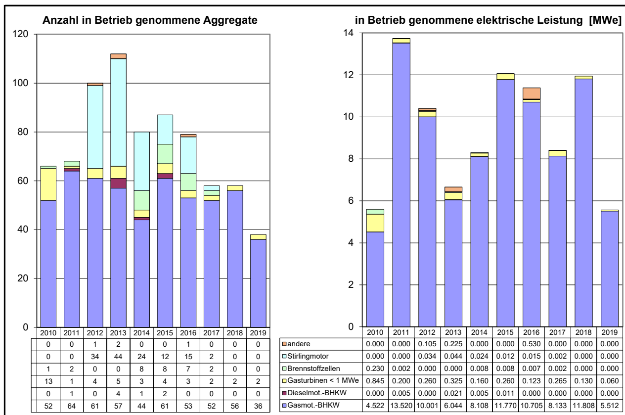
Bild 6.4c In Betrieb genommene Klein-WKK-Aggregate der letzten 10 Jahre
