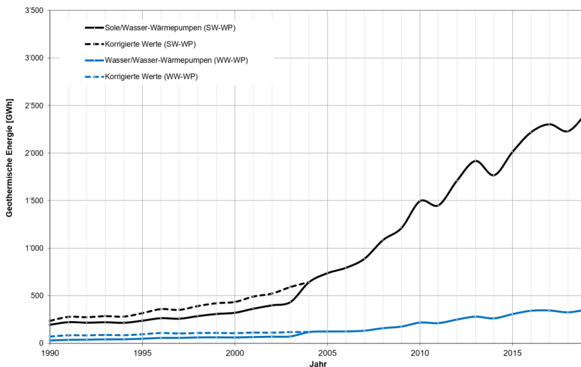
Figur 5: Entwicklung der gefördertener geothermischen (erneuerbaren) Energie für die SW-WP und für die auf geothermischer Nutzung basierenden WW-WP-Anlagen.
