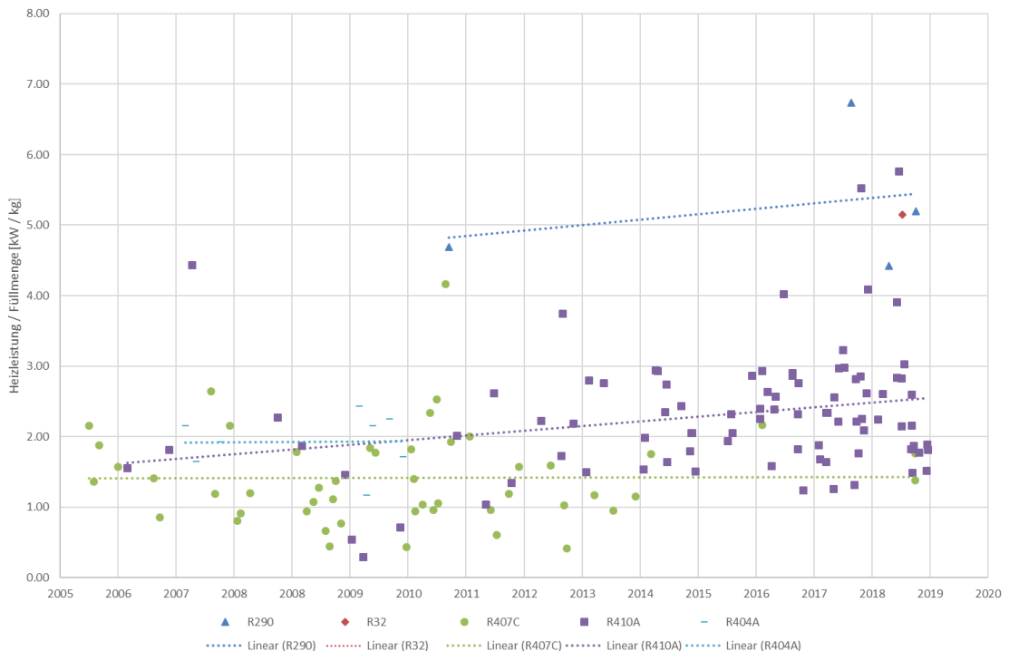
Abb. 1.6: Heizleistung pro Kältemittelfüllmenge bei Luft/Wasser-Wärmepumpen seit 2005
