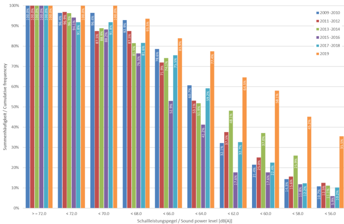
Abb. 1.8: Schalleistungspegelverteilung aller Wärmepumpentypen
