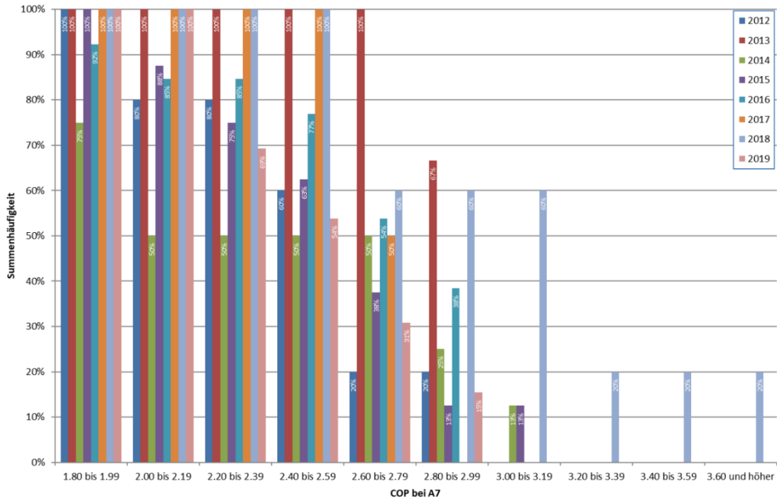
Abb. 2.2: COP-Verteilung aller geprüften Warmwasser-Wärmepumpen bei A7
