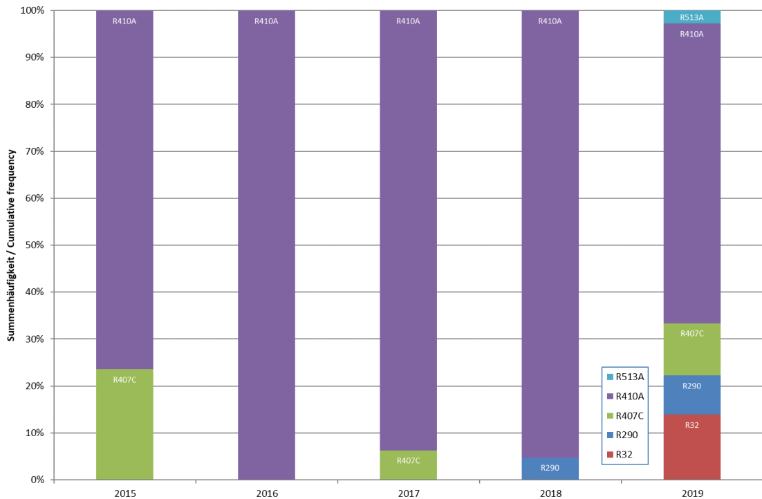
Abb. 1.5: verwendete Kältemitteltypen bei Luft/Wasser-Wärmepumpen seit 2015
