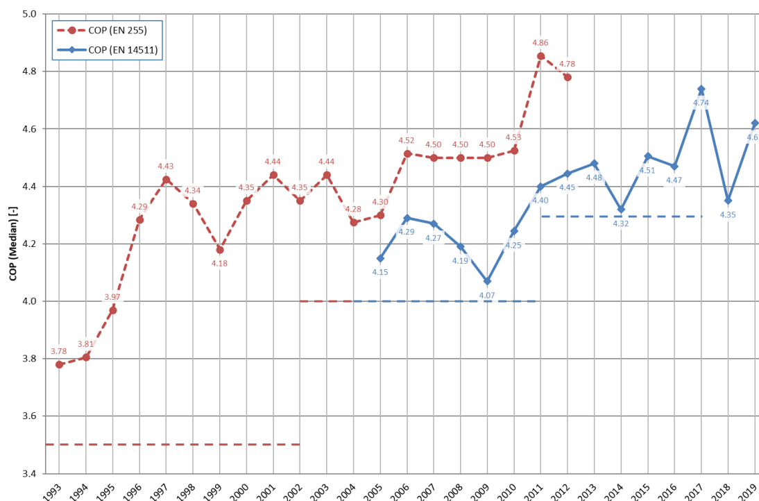
Abb. 1.9: COP-Entwicklung der Sole/Wasser-Wärmepumpe seit 1993
