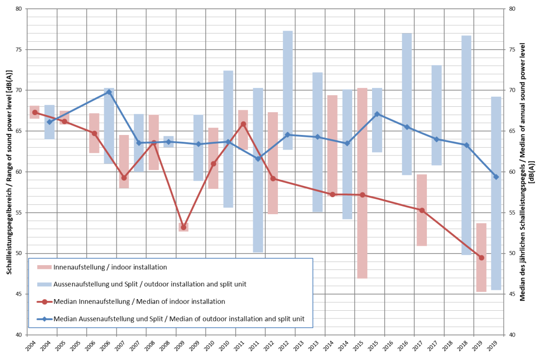
Abb. 1.7: Schalleistungspegelentwicklung zwischen Innenaufstellung und Aussenaufstellung / Split
