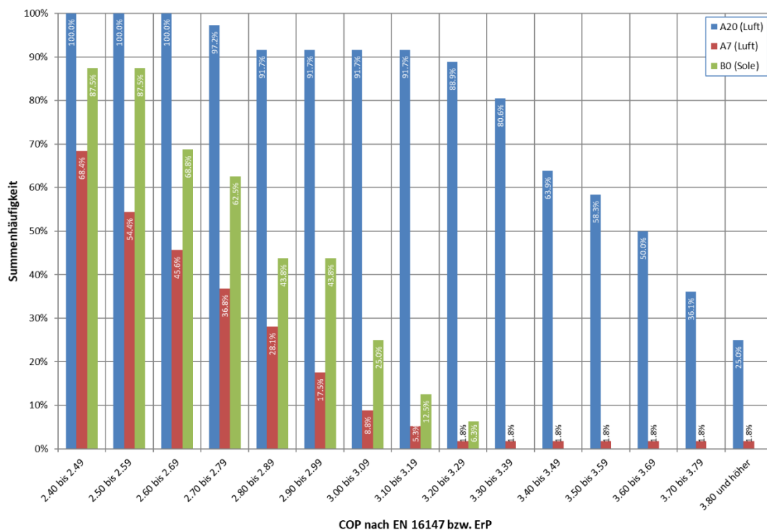
Abb. 2.1: COP-Verteilung aller geprüften Warmwasser-Wärmepumpen nach EN 16147
