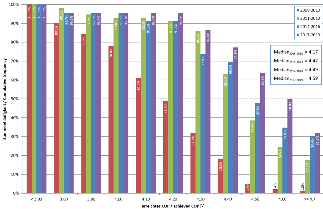
Abb. 1.10: COP-Verteilung in der zeitlichen Entwicklung
