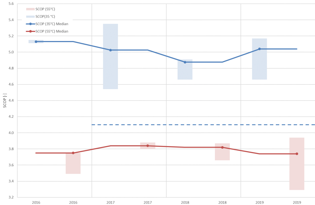
Abb. 1.11: SCOP-Entwicklung der Sole/Wasser-Wärmepumpen
