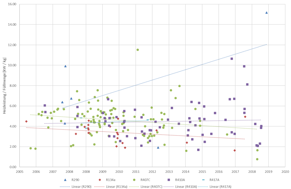
Abb. 1.13: Heizleistung pro Kältemittelfüllmenge bei Sole/Wasser-Wärmepumpen seit 2005
