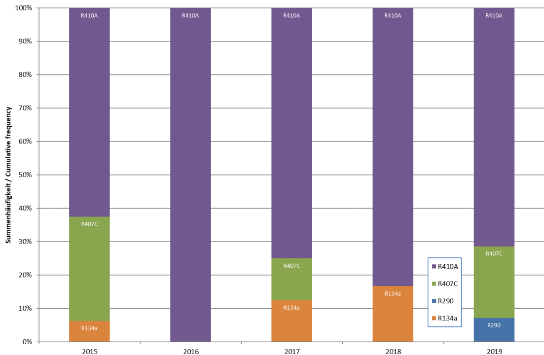
Abb. 1.12: verwendete Kältemitteltypen bei Sole/Wasser-Wärmepumpen seit 2015
