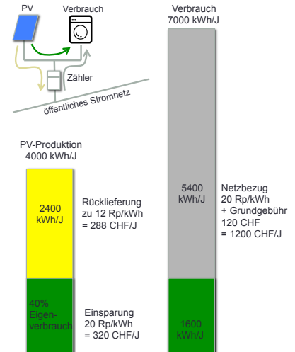
Abbildung 3: 4kWp Anlage-Beispiel B
